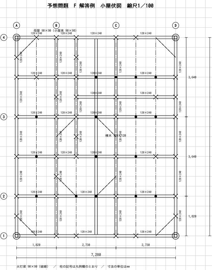
(4) 小屋伏図 (1/100)
