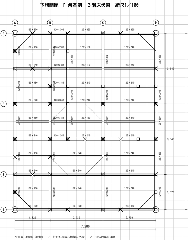
(4) 3階床伏図 (1/100)
