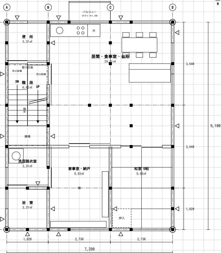
(2) 2階平面図 縮尺1/100
