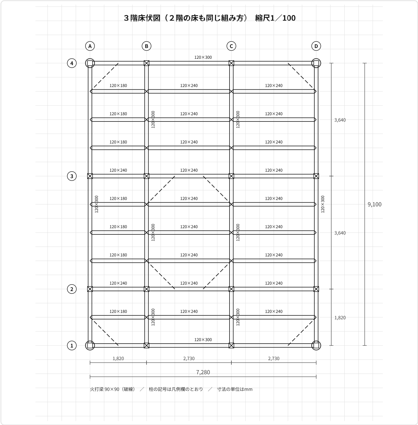
床伏図。線1本1本が木の棒で、その太さが書きこんである。
