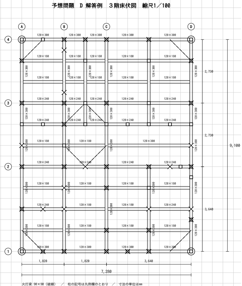
(4) 3階床伏図
