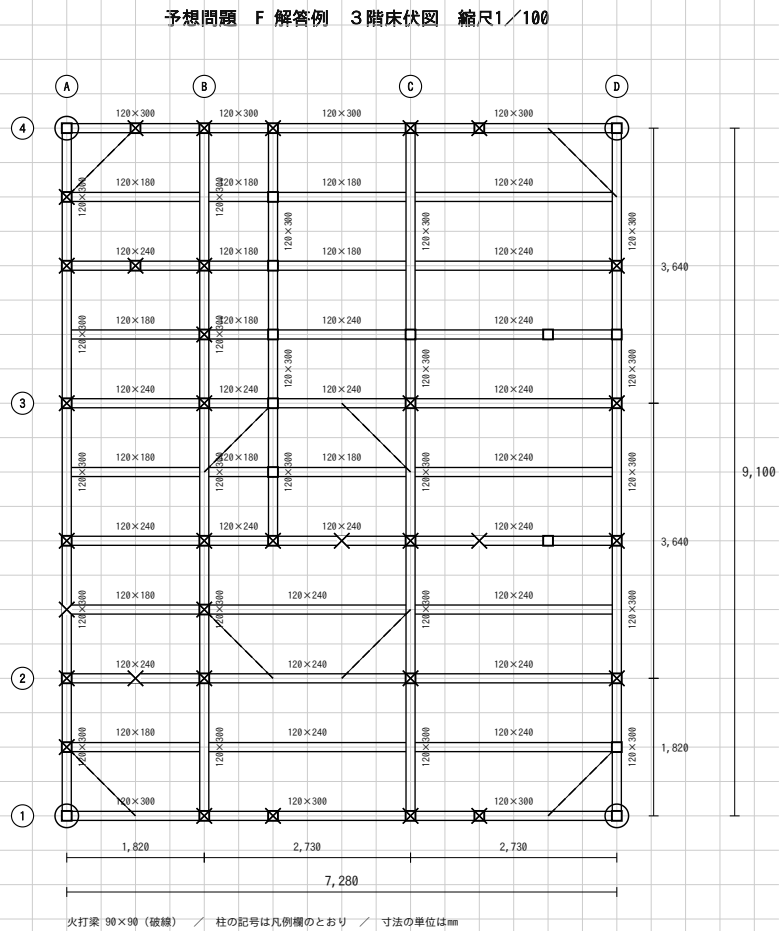
(4) 3階床伏図
