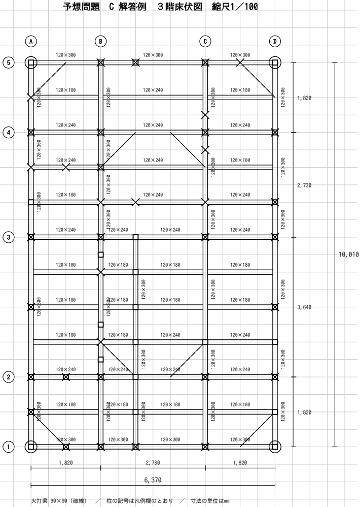
(4) 3階床伏図
