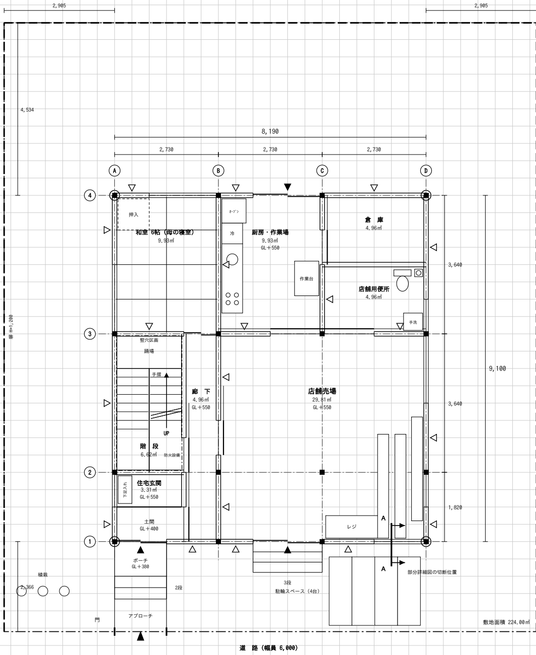
(1) 1階平面図 兼 配置図 縮尺1／100 (目盛4.55mm)
