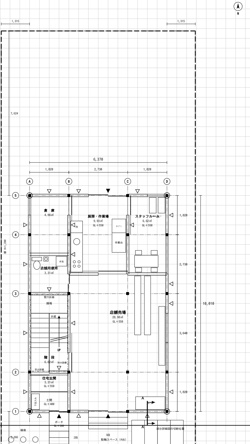
(1) 1階平面図 兼 配置図 縮尺1／100 (目盛4.55mm)
