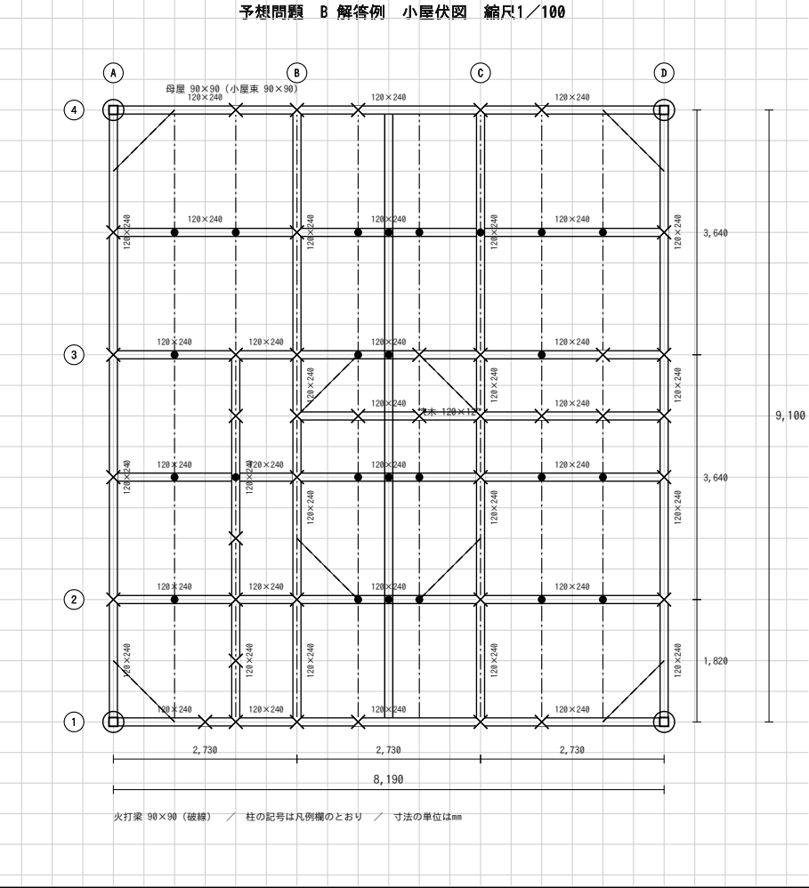
(4) 小屋伏図
