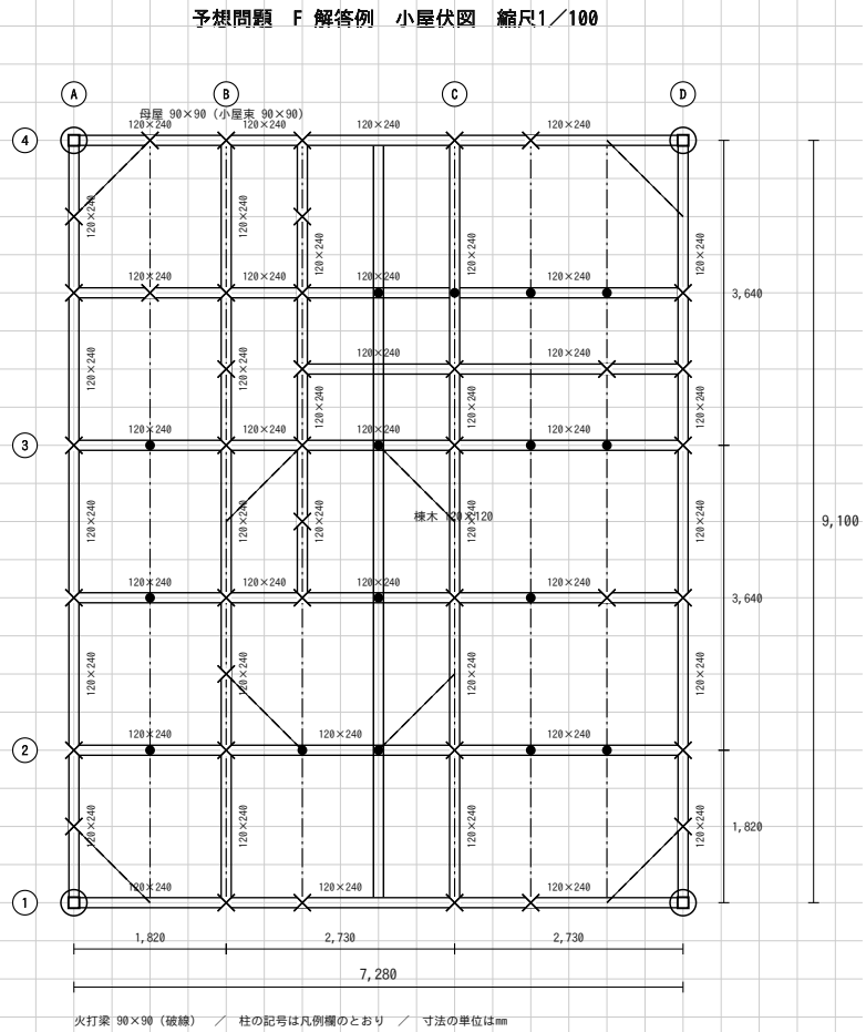
(4) 小屋伏図
