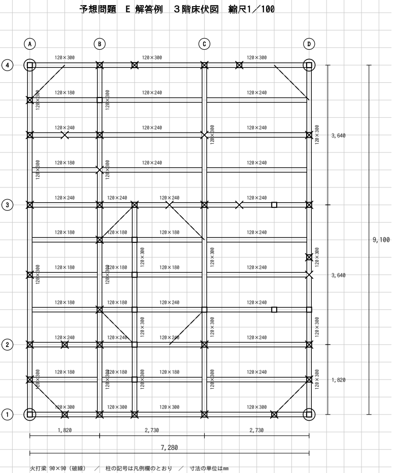
(4) 3階床伏図
