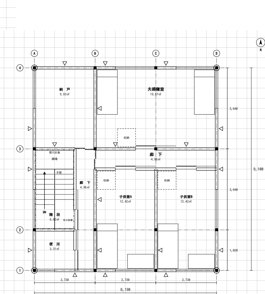
(3) 3階平面図 縮尺1／100 (目盛4.55mm)
