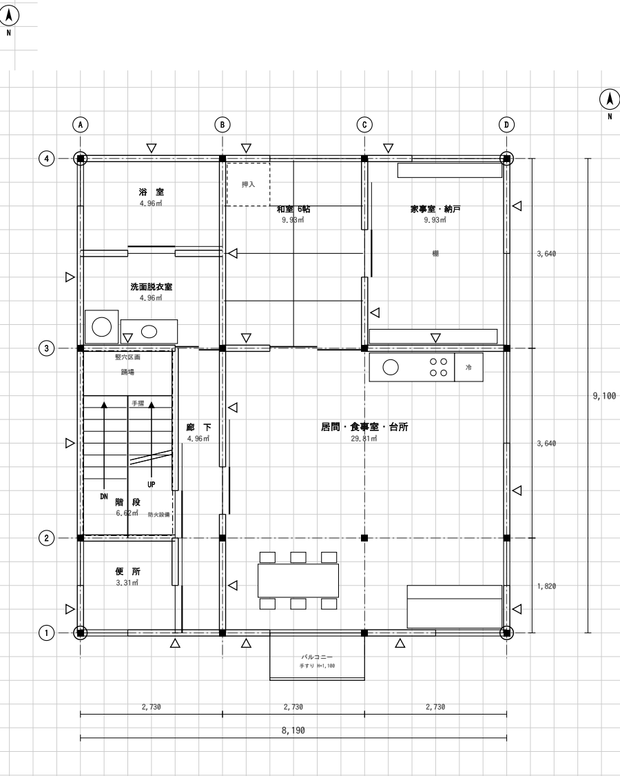
(2) 2階平面図 縮尺1／100 (目盛4.55mm)
