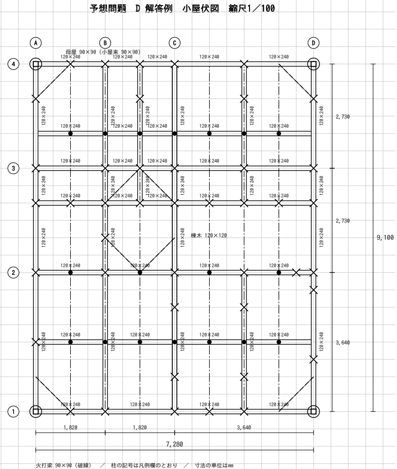
(4) 小屋伏図
