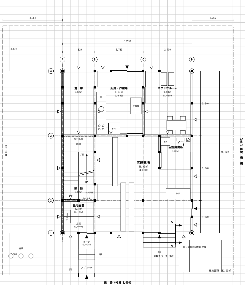
(1) 1階平面図 兼 配置図 縮尺1／100 (目盛4.55mm)
