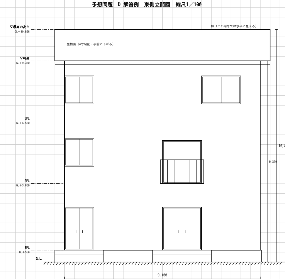
(5) 東側立面図
