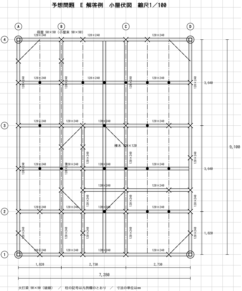
(4) 小屋伏図
