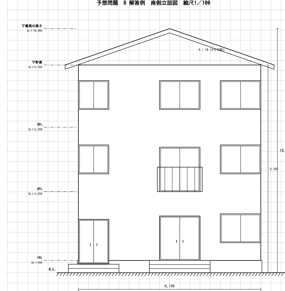
(5) 南側立面図
