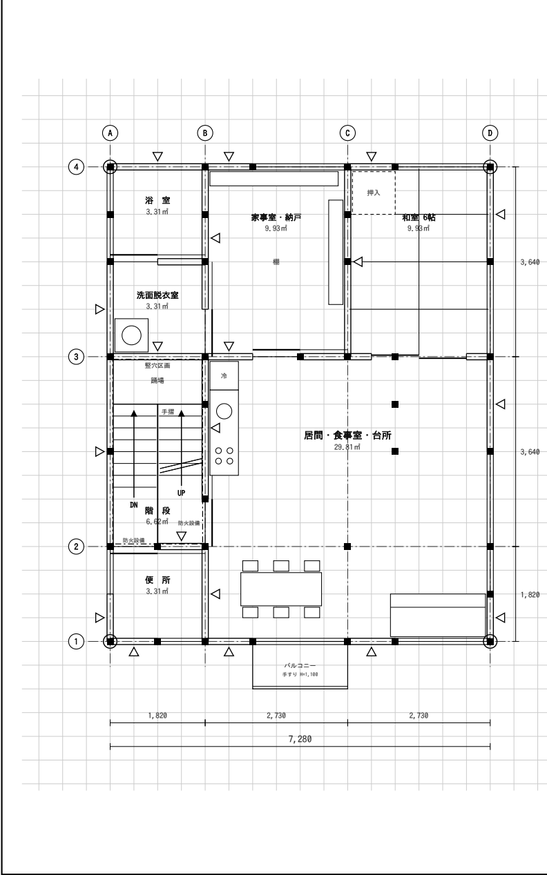
(3) 3階平面図 縮尺1／100 (目盛4.55mm)
