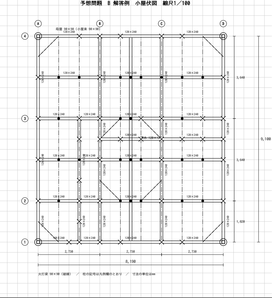
(4) 小屋伏図
