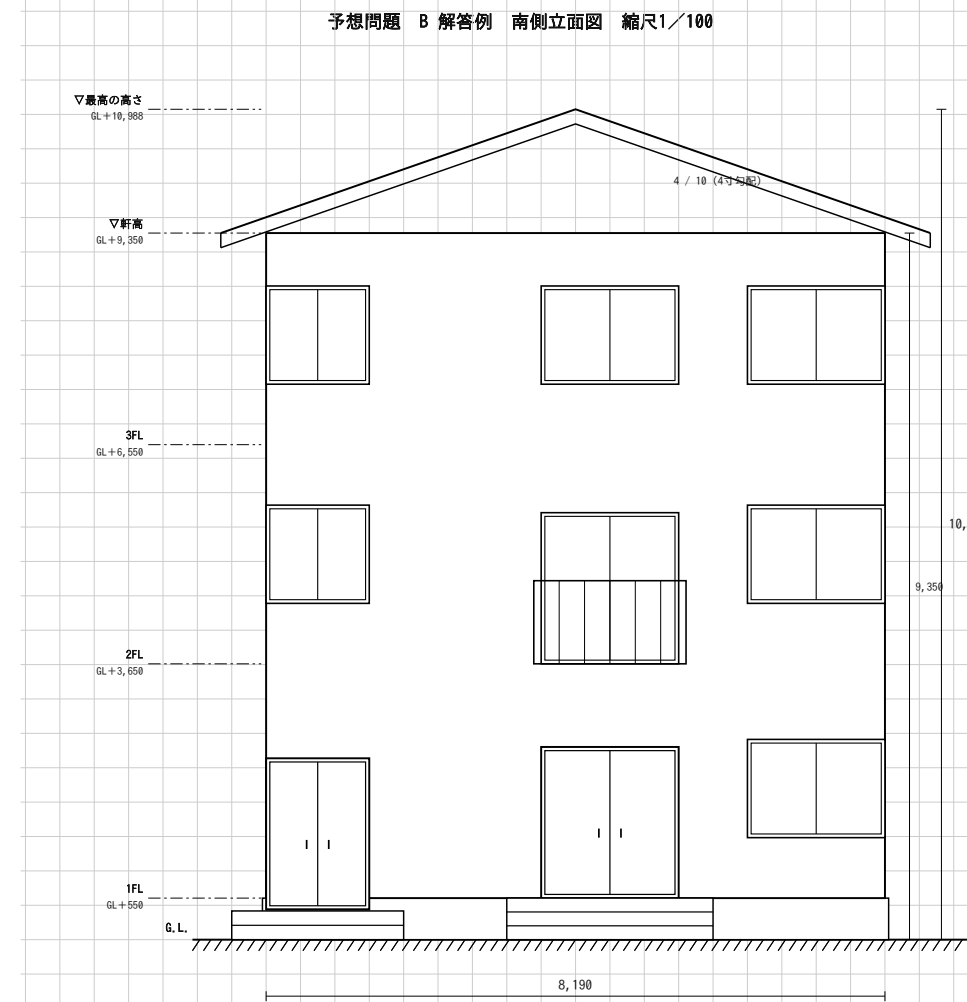
(5) 南側立面図
