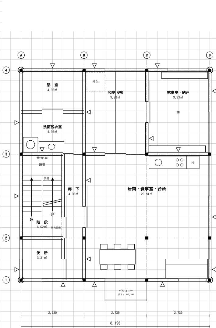
(2) 2階平面図 縮尺1／100 (目盛4.55mm)
