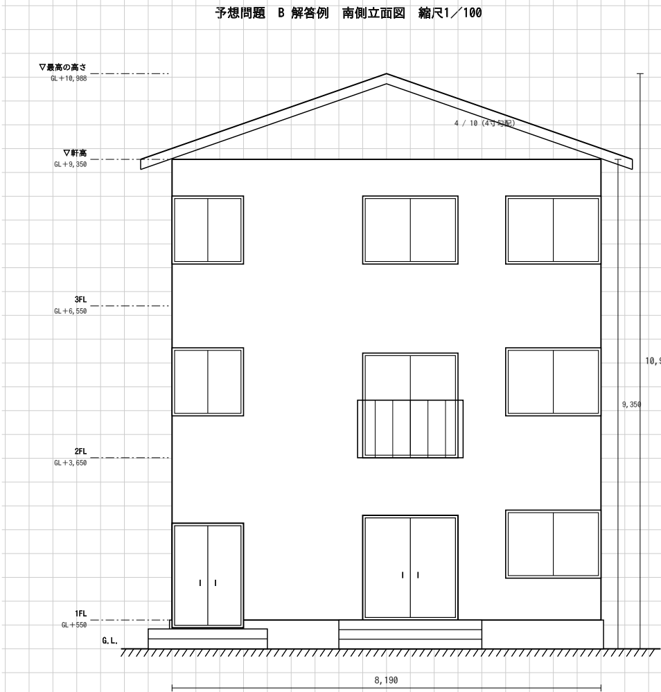
(5) 南側立面図
