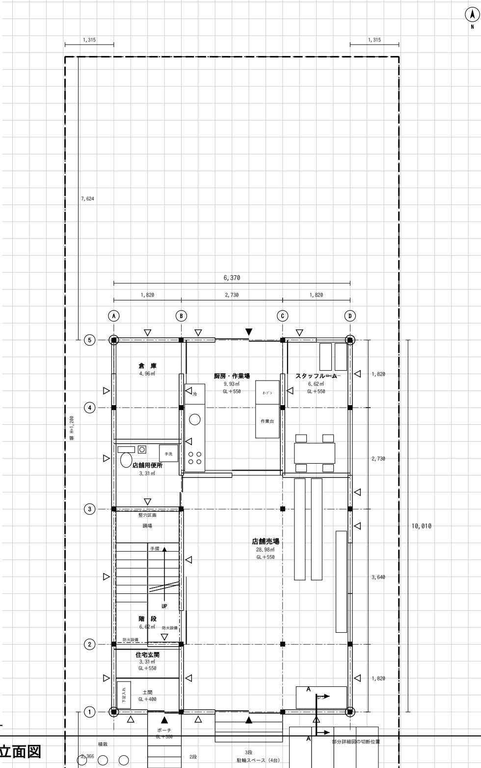
(1) 1階平面図 兼 配置図 縮尺1／100 (目盛4.55mm)
