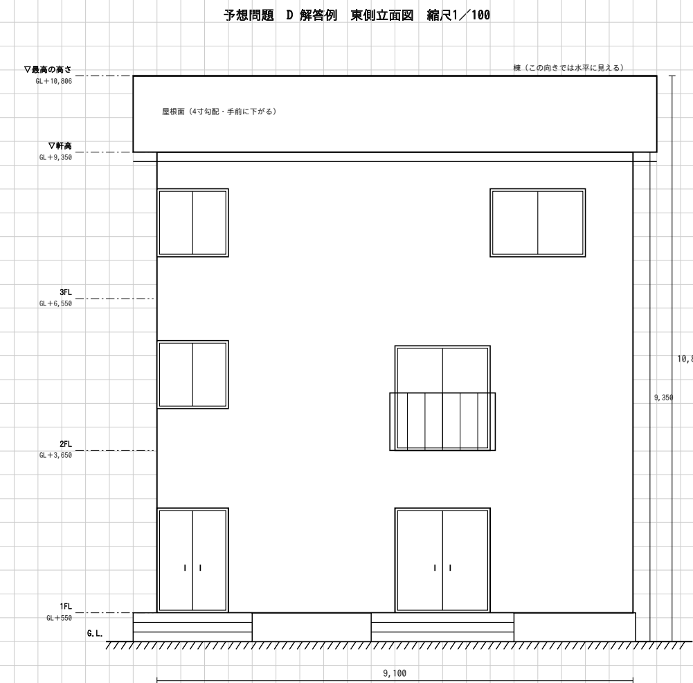
(5) 東側立面図
