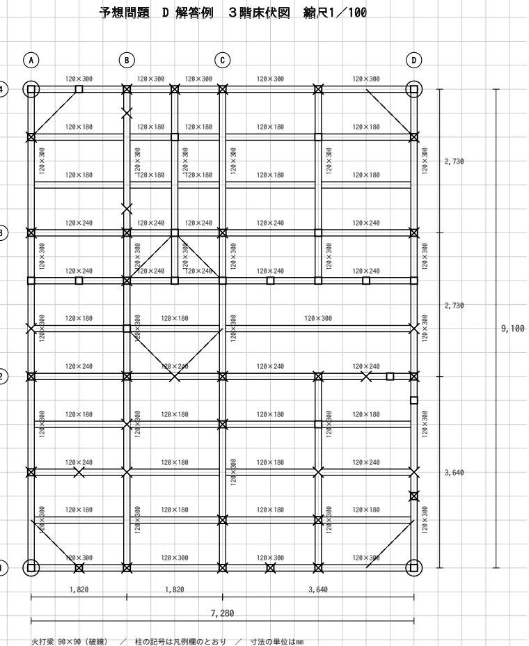
(4) 3階床伏図
