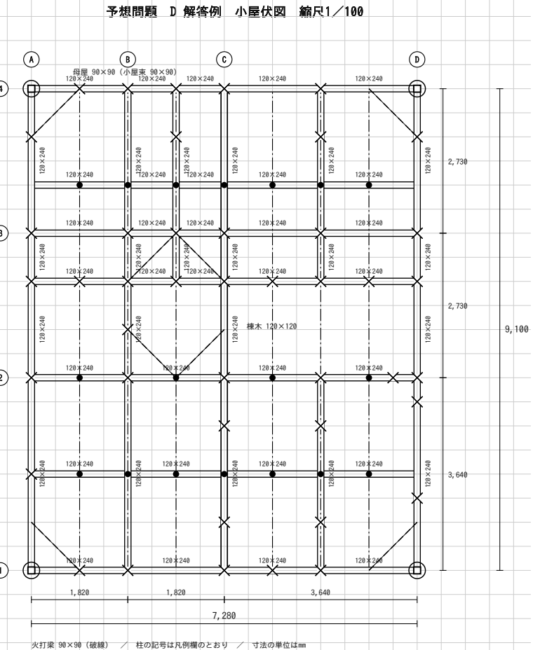
(4) 小屋伏図
