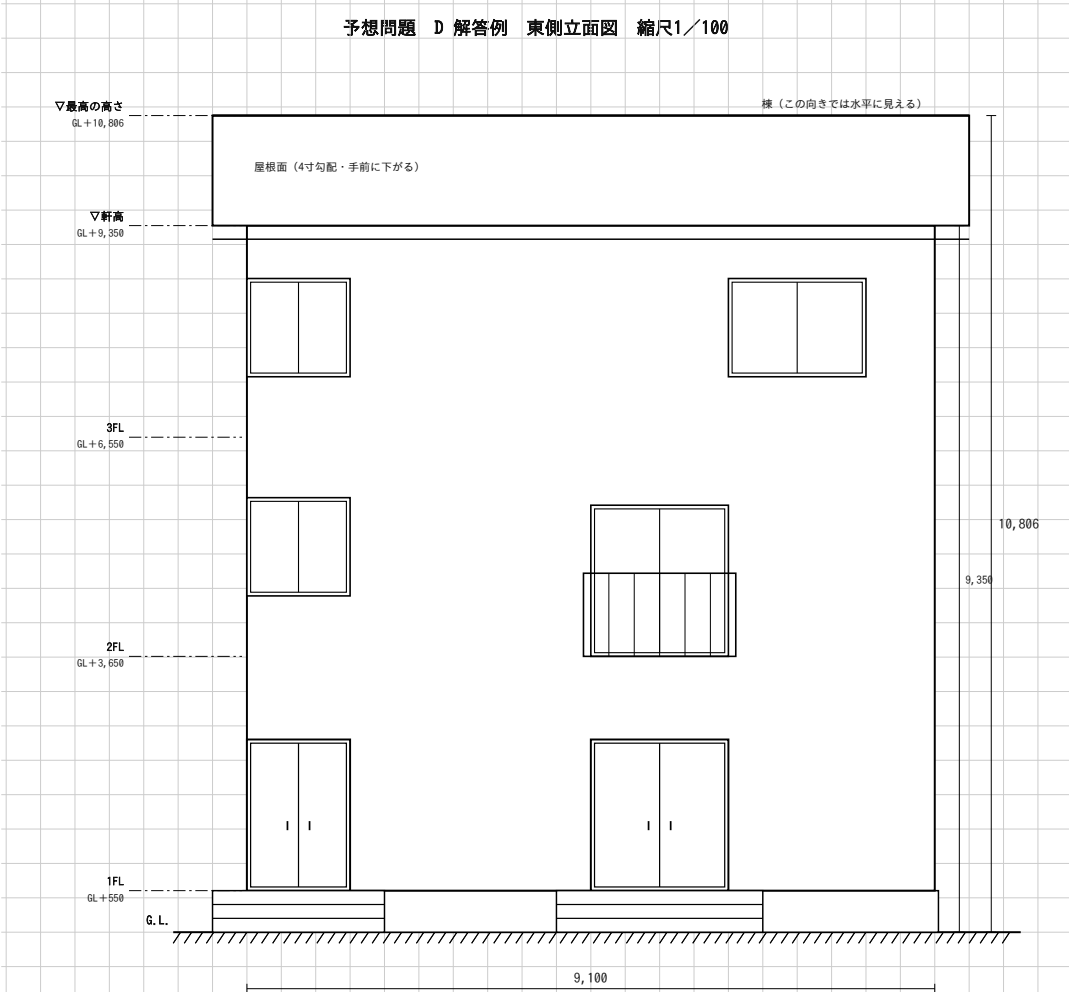
(5) 東側立面図
