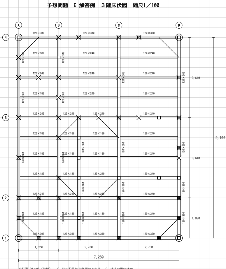
(4) 3階床伏図
