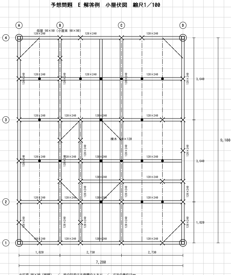
(4) 小屋伏図
