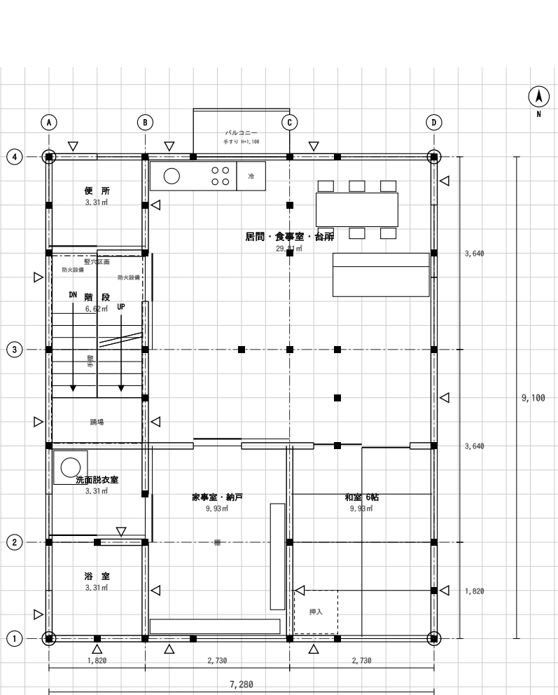
(2) 2階平面図 縮尺1／100 (目盛4.55mm)
