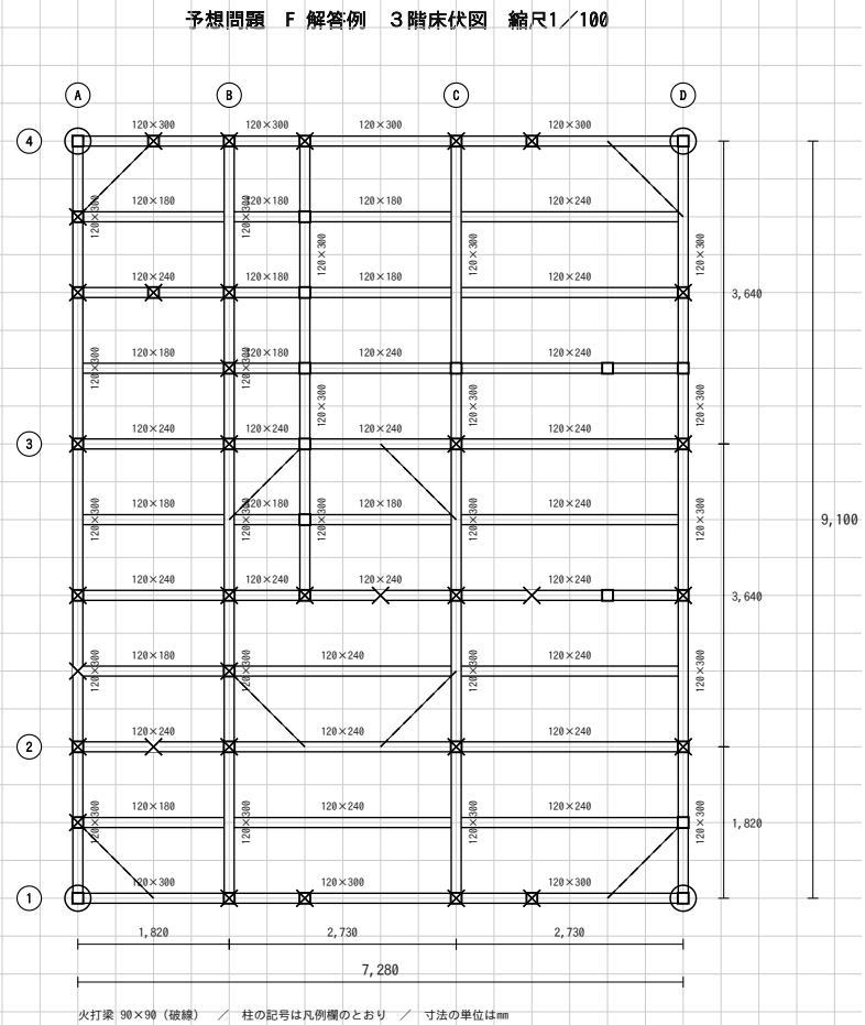
(4) 3階床伏図
