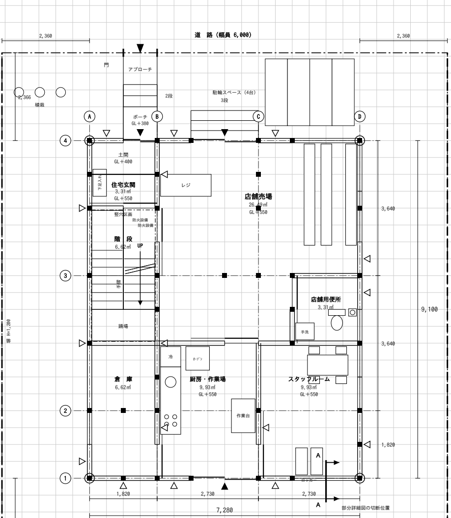
(1) 1階平面図 兼 配置図 縮尺1／100 (目盛4.55mm)
