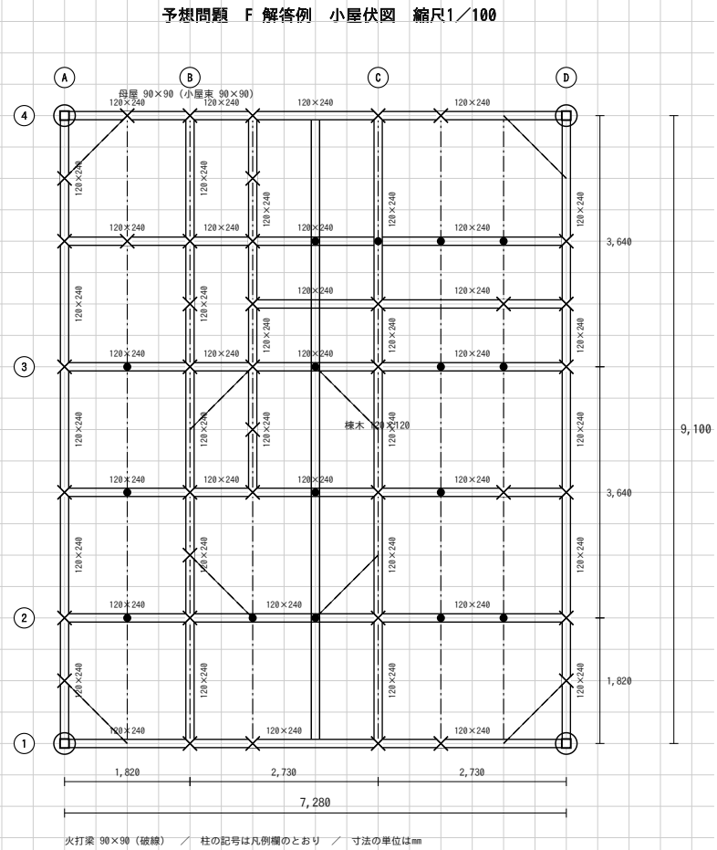
(4) 小屋伏図
