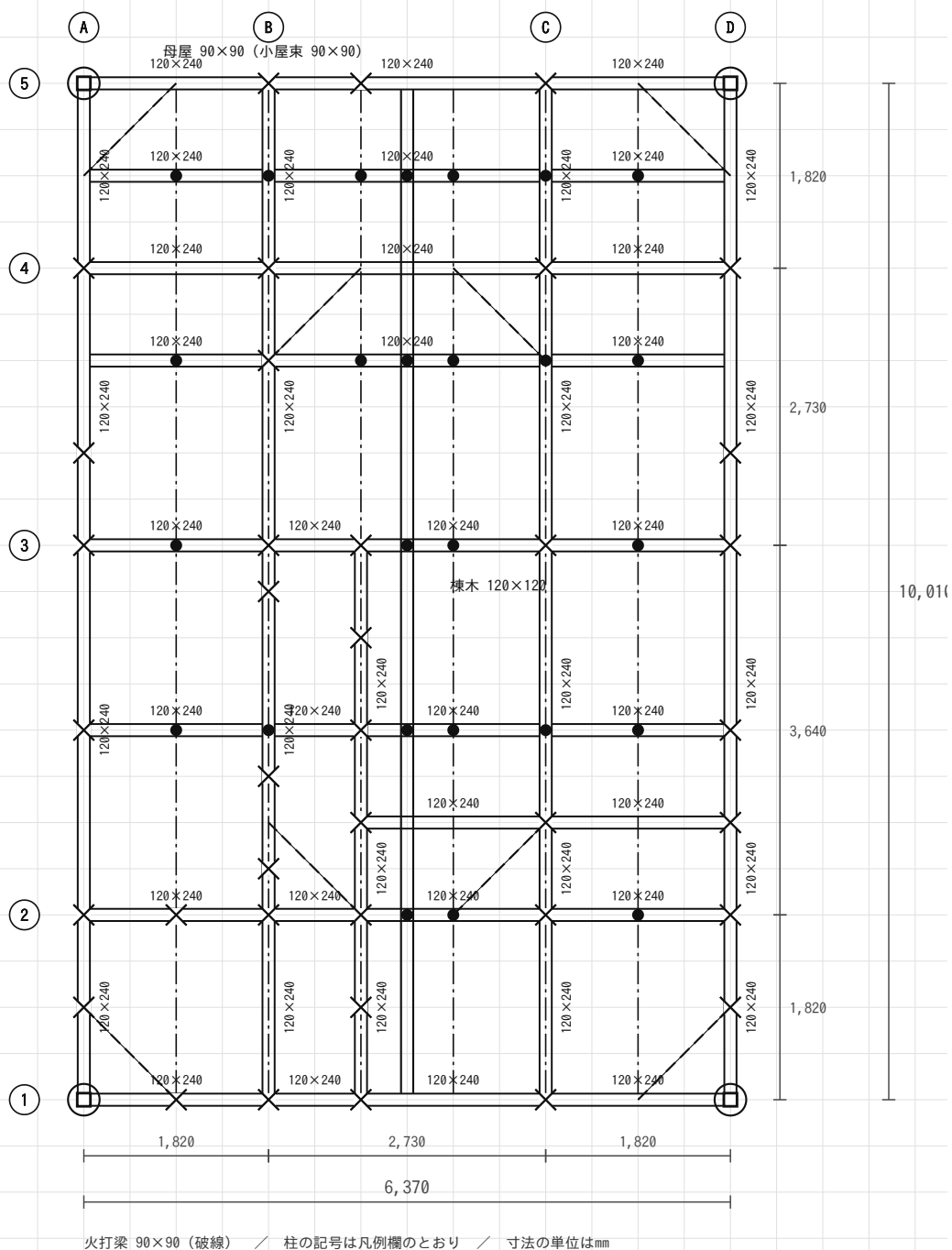
予想問題 C 解答例 小屋伏図 縮尺1/100
