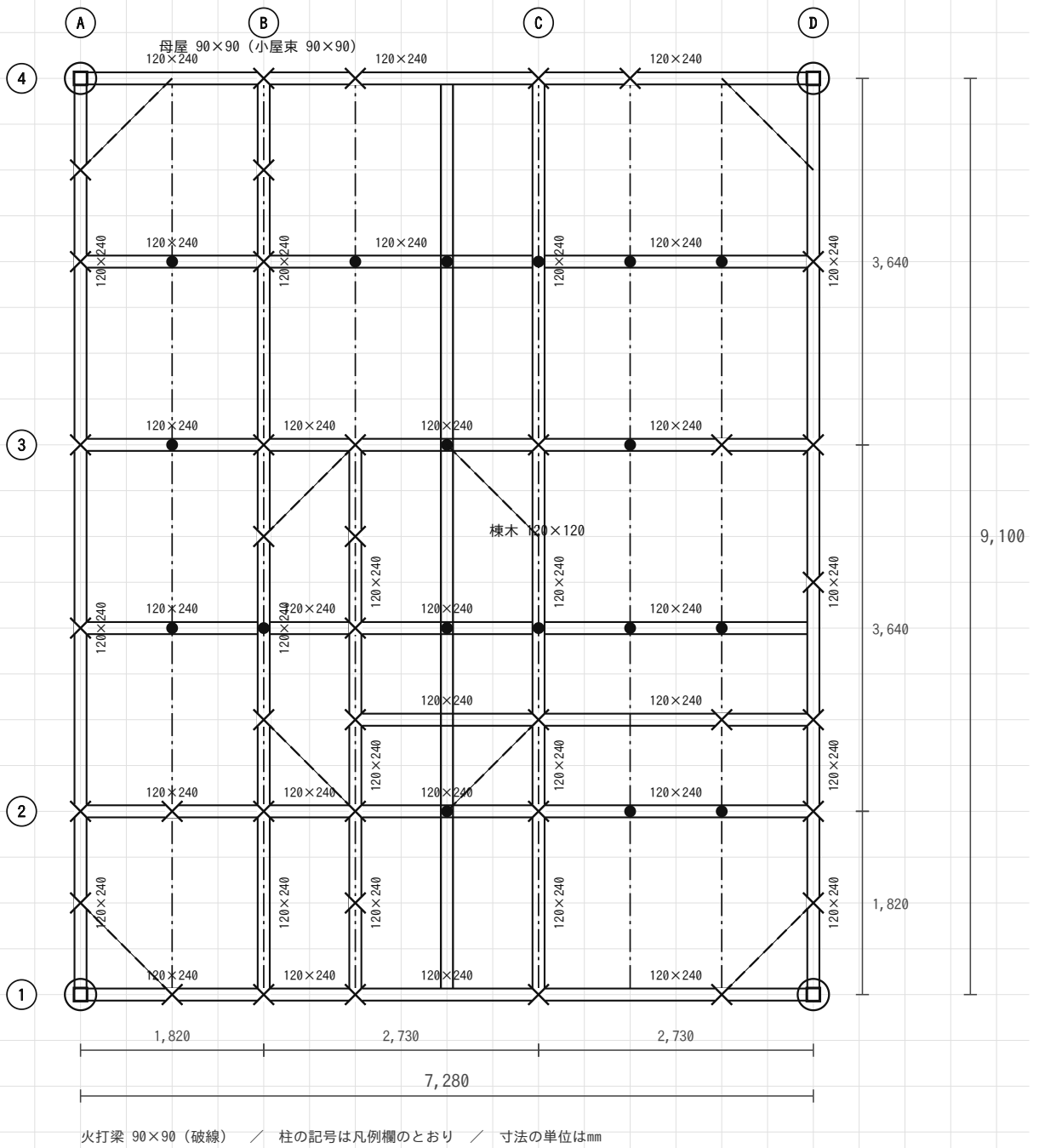
予想問題 E 解答例 小屋伏図 縮尺1/100
