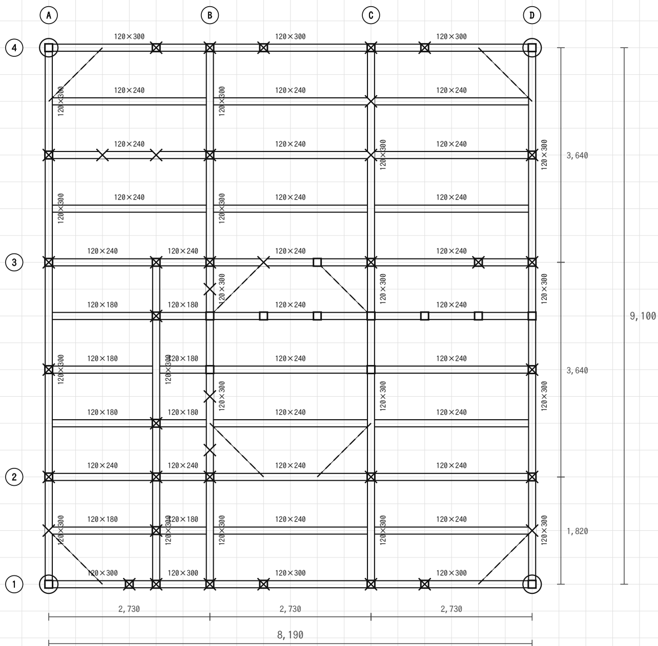
予想問題 B 解答例 3階床伏図 縮尺1/100
