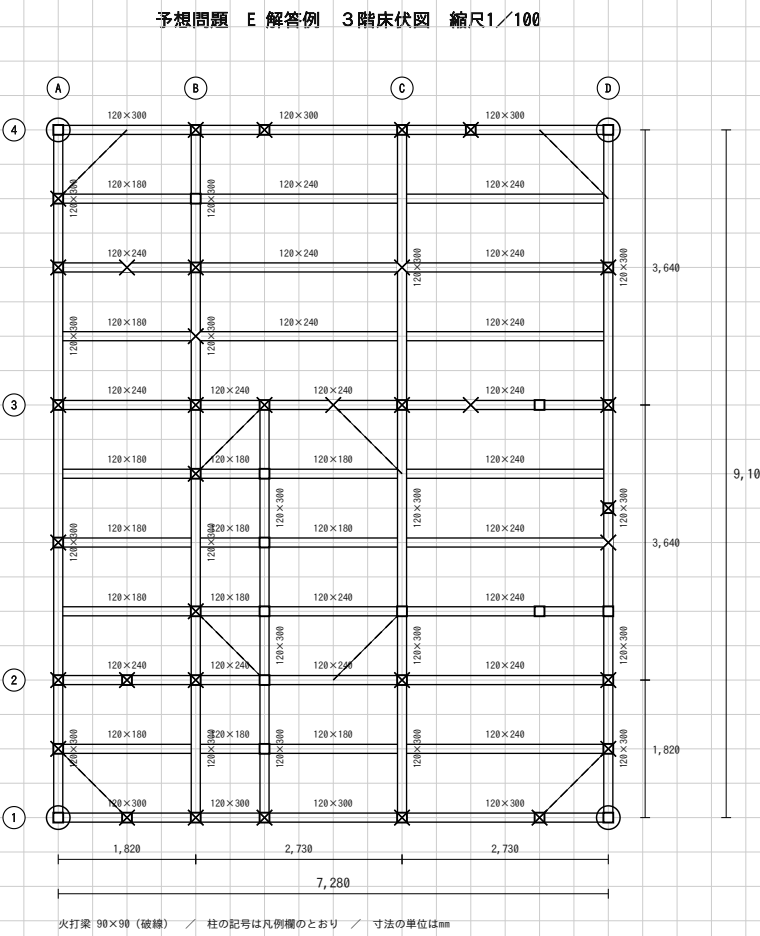
(4) 3階床伏図 (1/100)
