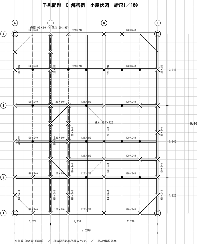
(4) 小屋伏図 (1/100)
