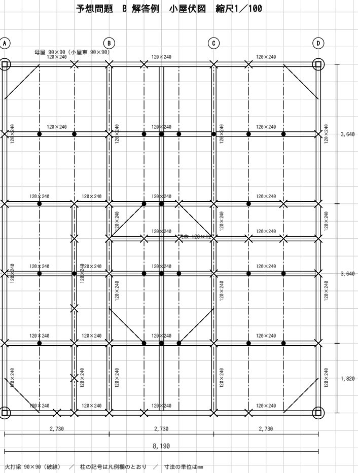
(4) 小屋伏図 (1/100)
