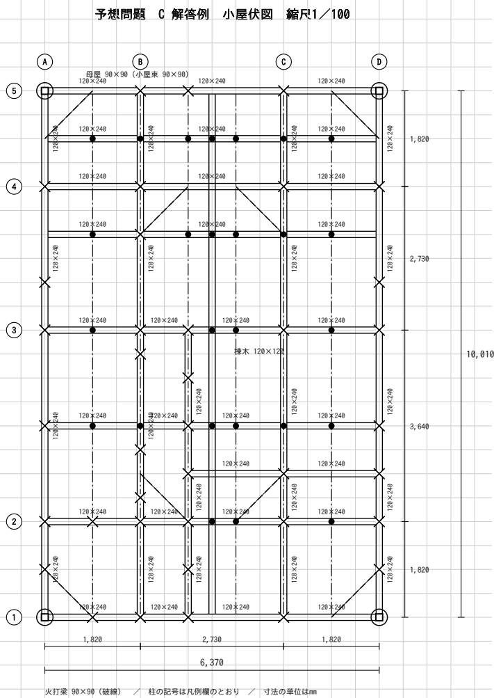
(4) 小屋伏図 (1/100)
