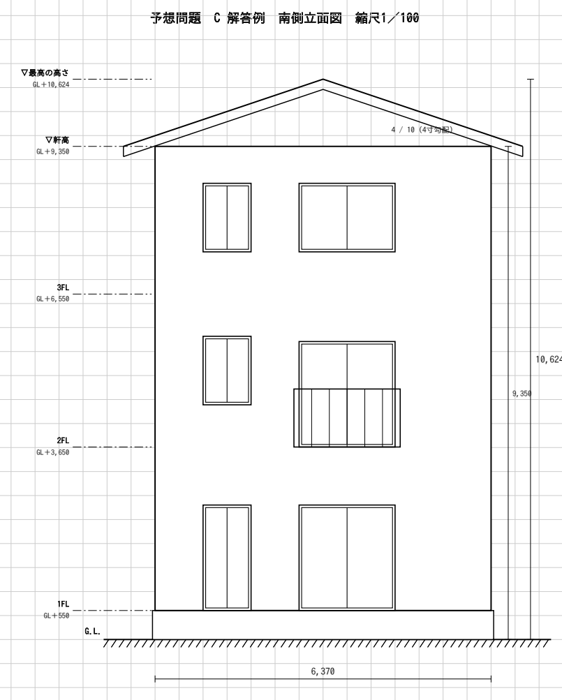
(5) 南側立面図 (1/100)
