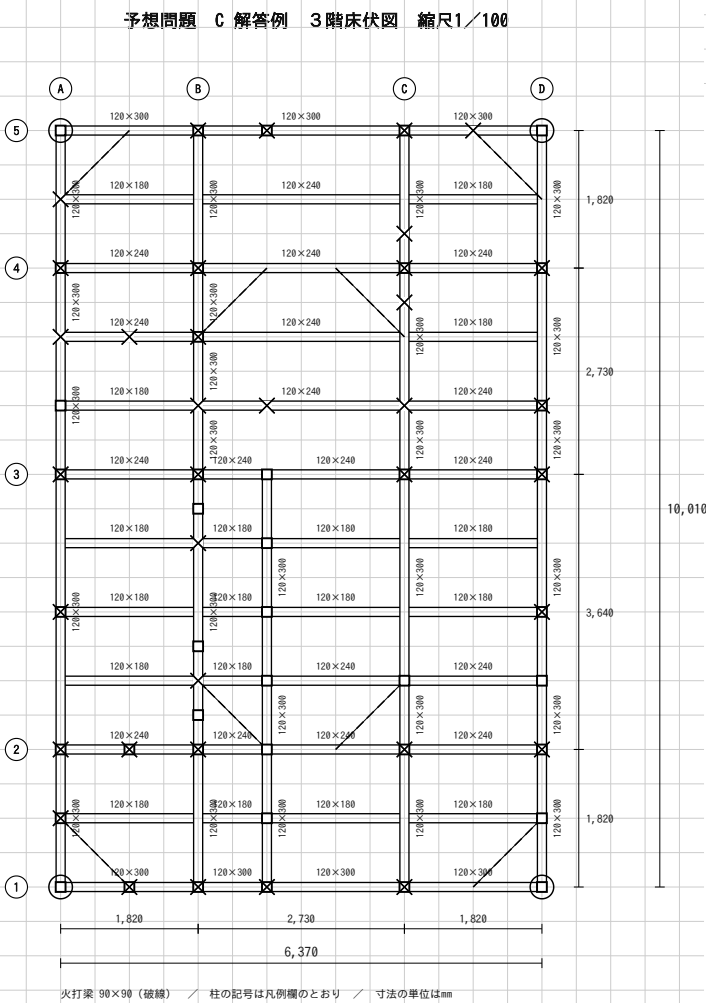
(4) 3階床伏図 (1/100)
