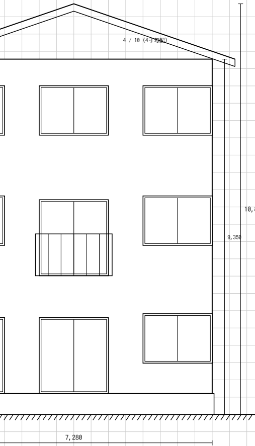
南側立面図 縮尺1/100
