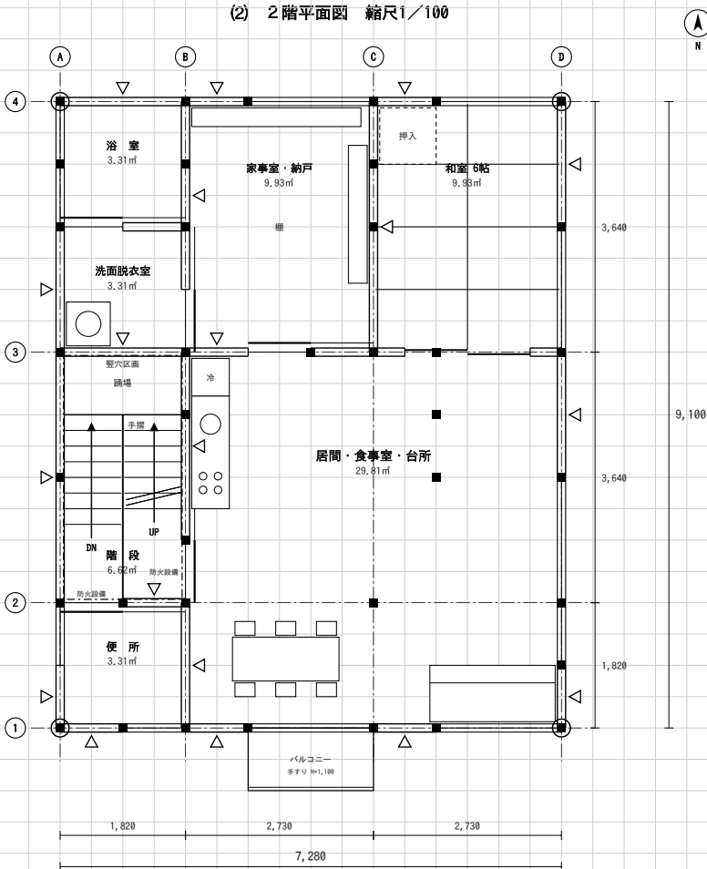
(2) 2階平面図 縮尺1/100
