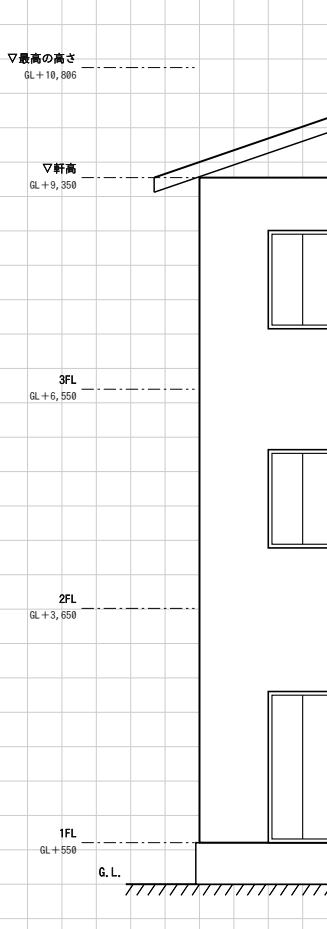
(5) 南側立面図 (1/100)
