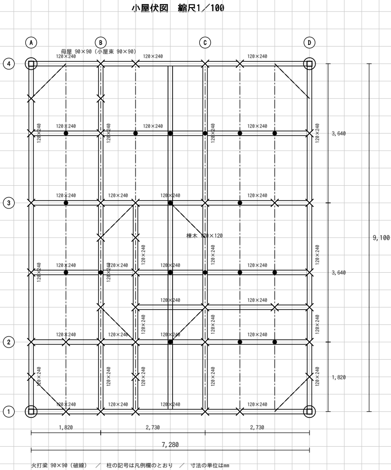
(4) 小屋伏図 (1/100)
