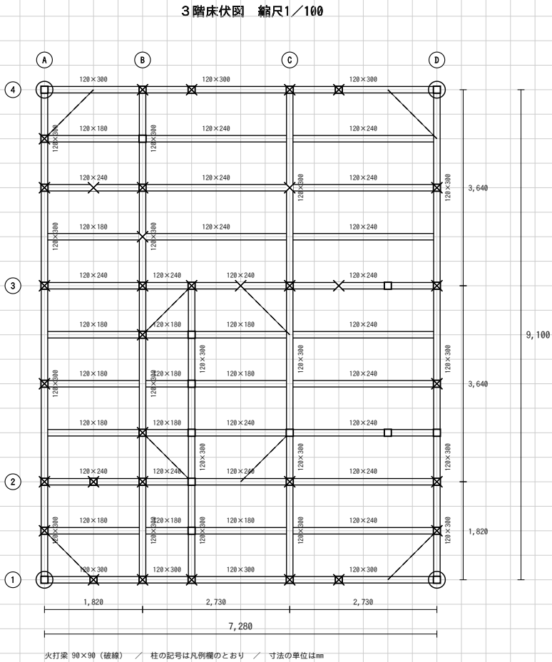
(4) 3階床伏図 (1/100)
