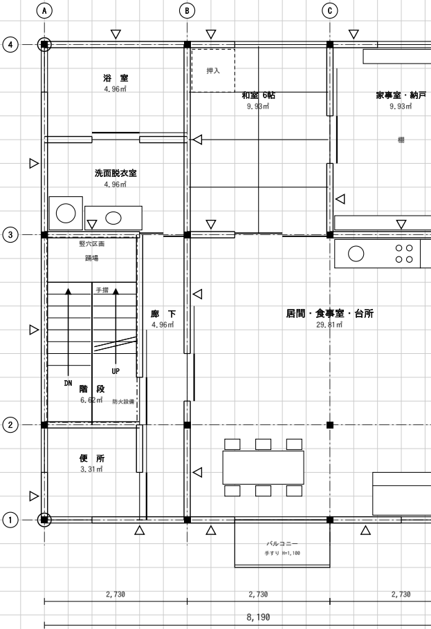
(2) 2階平面図 縮尺1/100
