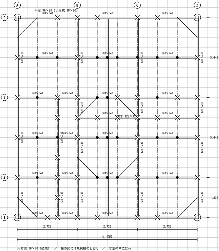
予想問題 B 解答例 小屋伏図 縮尺1/100
