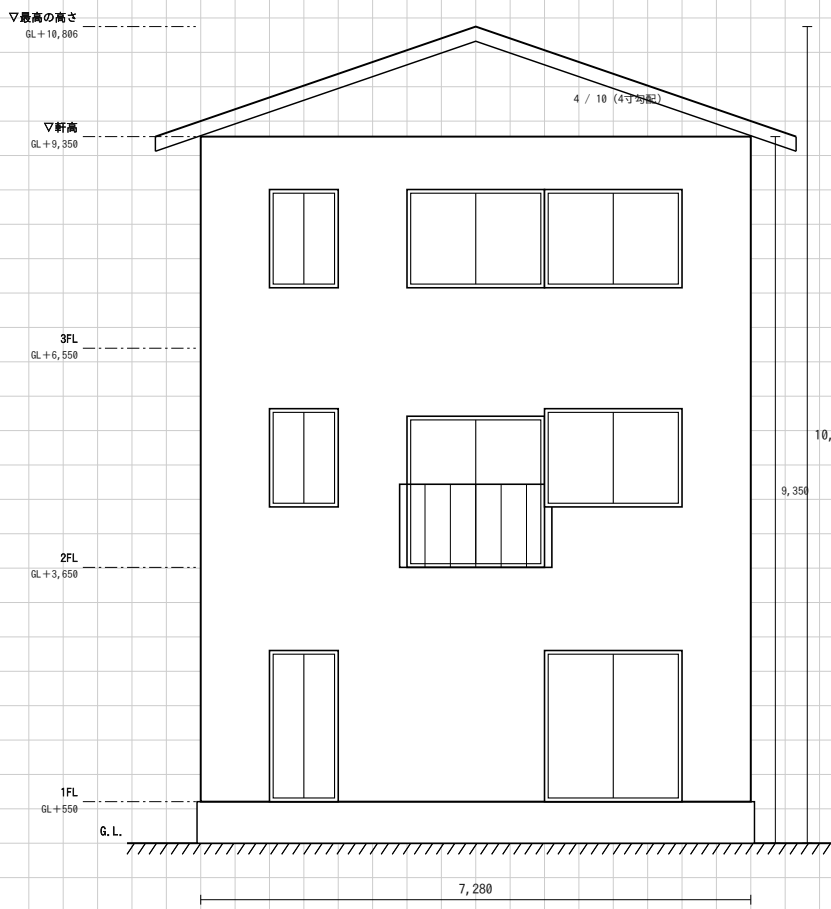
予想問題 E 解答例 南側立面図 縮尺1/100
