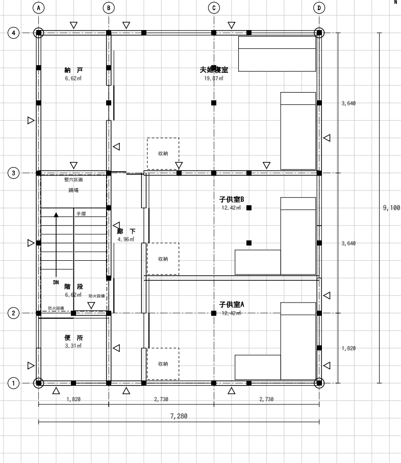
(3) 3階平面図 縮尺1/100
