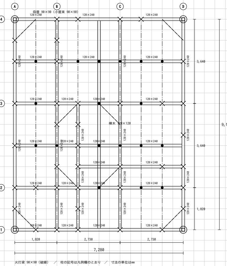
予想問題 E 解答例 小屋伏図 縮尺1/100
