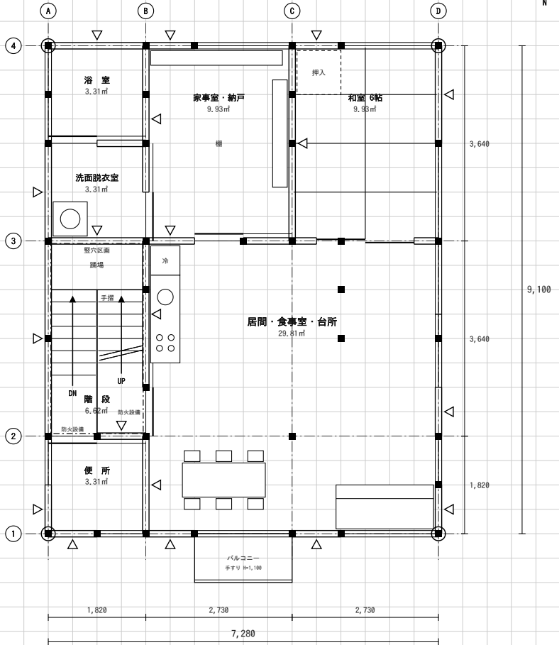
(2) 2階平面図 縮尺1/100
