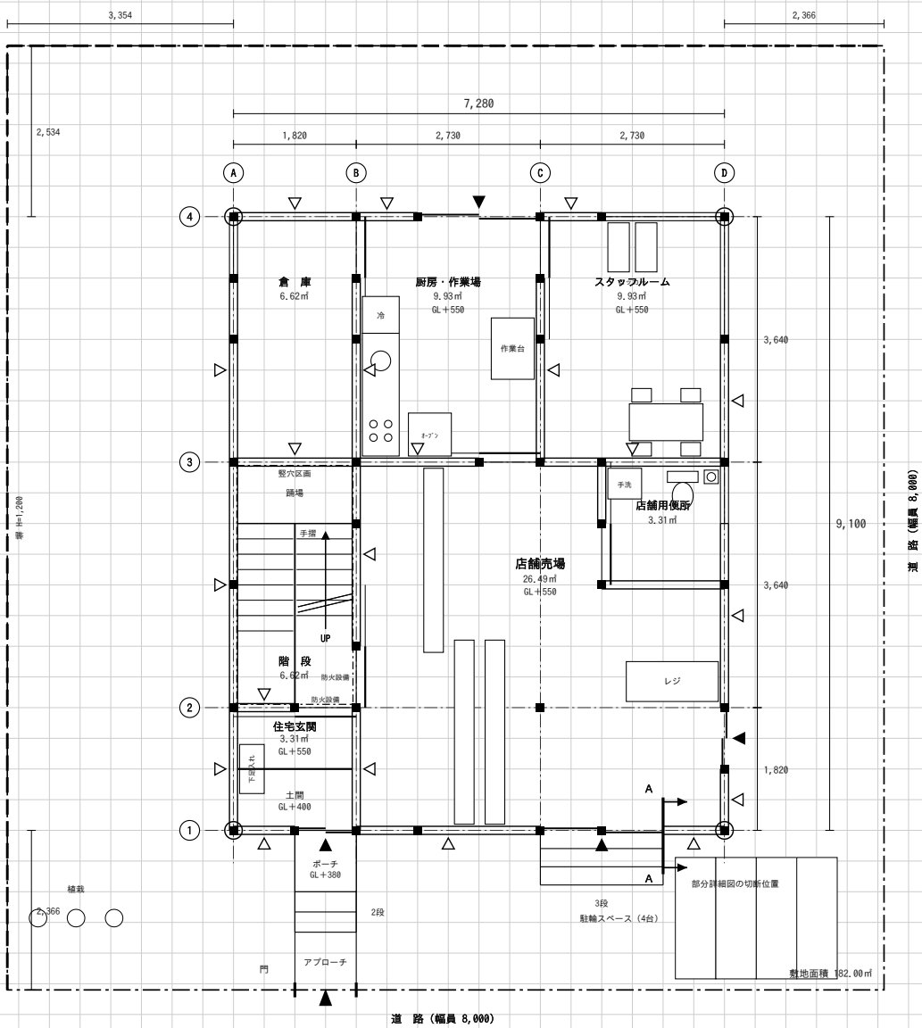
(1) 1階平面図 兼 配置図 縮尺1/100
