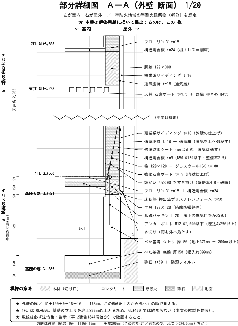
(6) 部分詳細図 (縦断面) (1/20)
