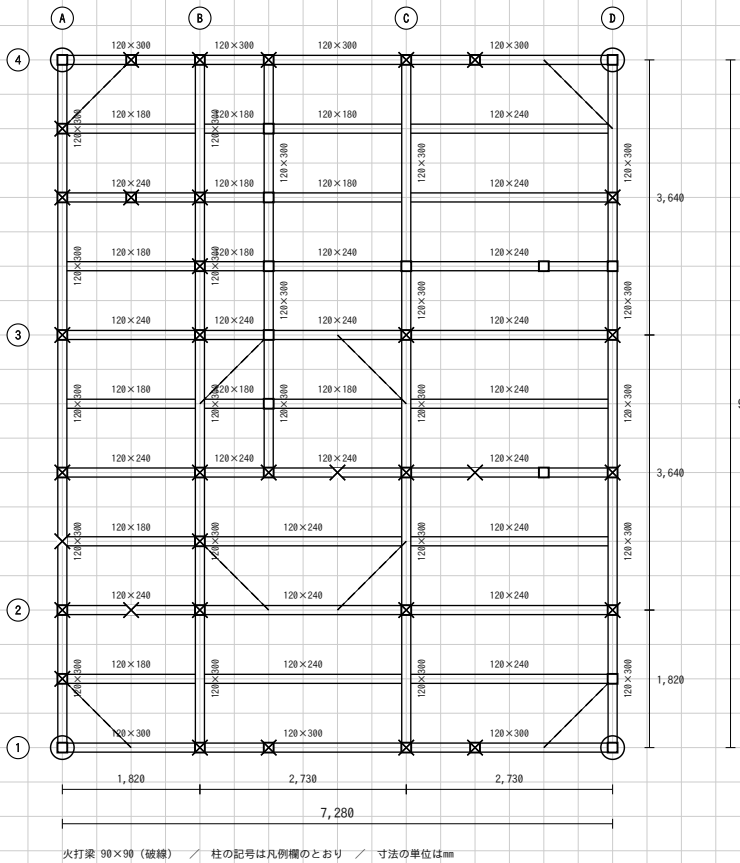
予想問題 F 解答例 3階床伏図 縮尺1/100
