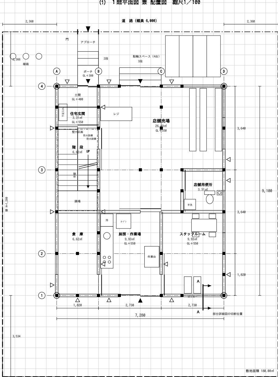
(1) 1階平面図 兼 配置図 縮尺1/100
