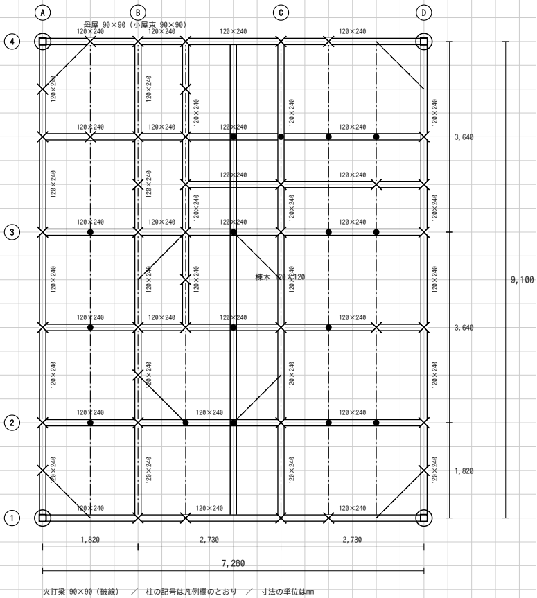
予想問題 F 解答例 小屋伏図 縮尺1/100
