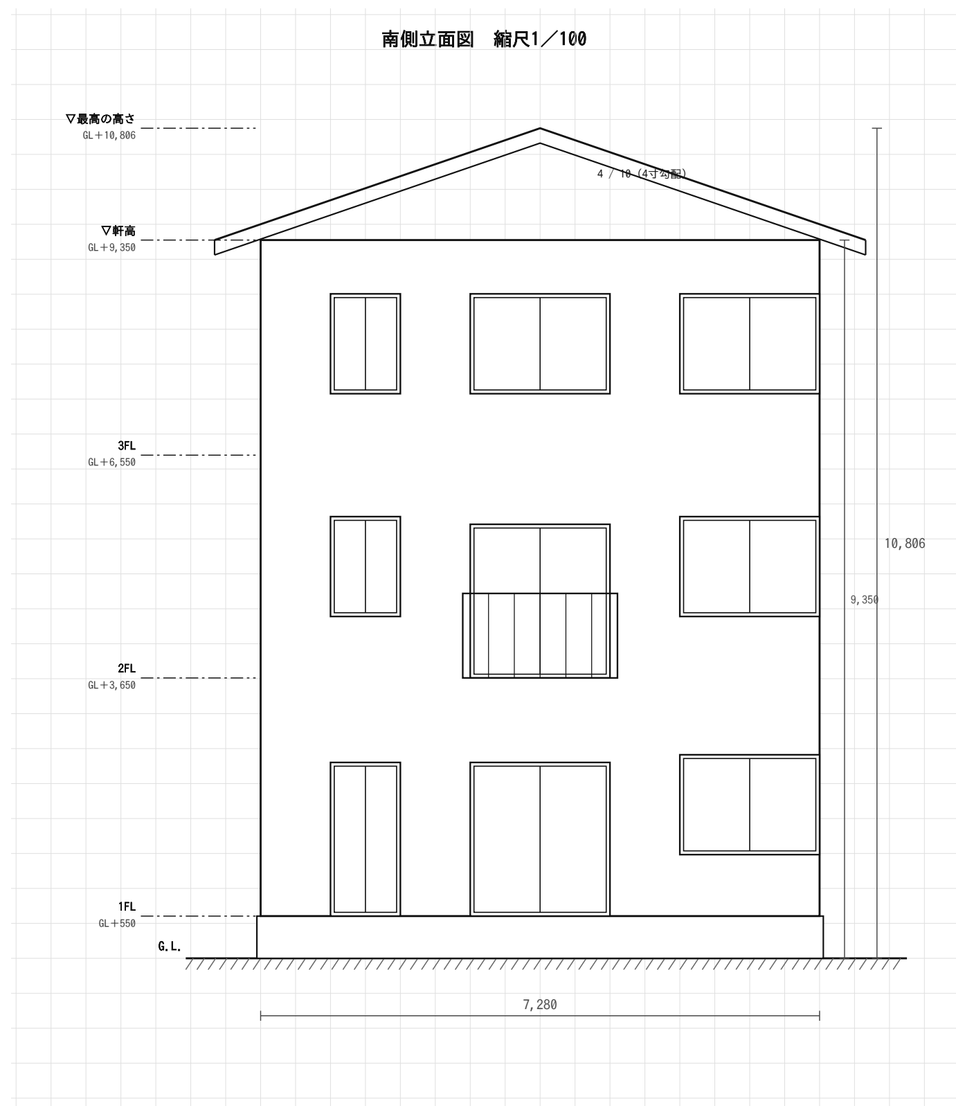
(5) 南側立面図 (1/100)
