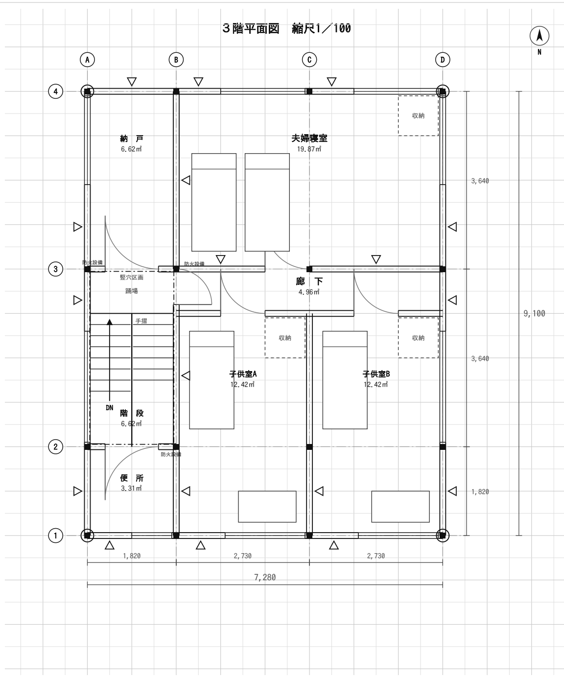
3階平面図。廊下を東西に1本通して、階段から全部の部屋へドアで入れるようにする。
