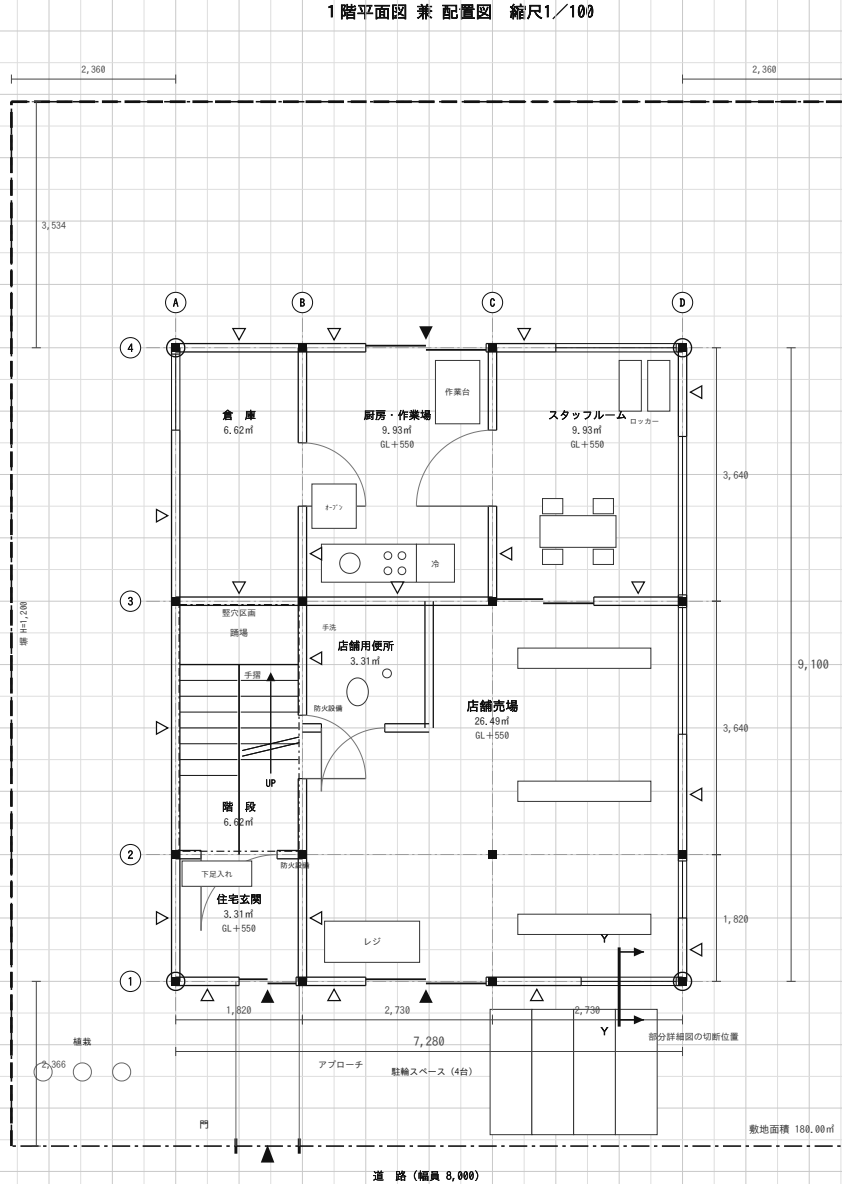
1階平面図 兼 配置図 縮尺1/100
