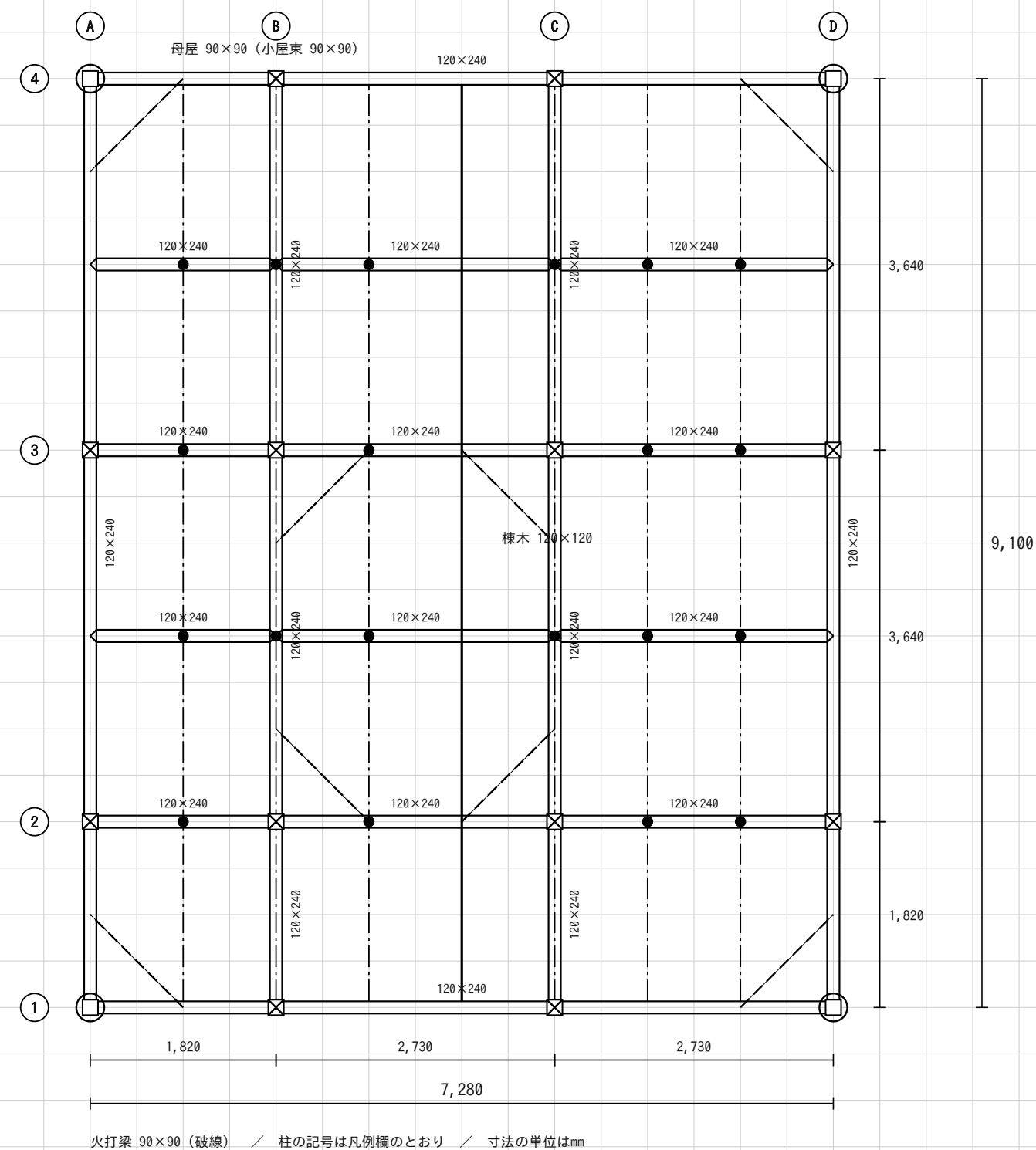
小屋伏図 縮尺1/100
