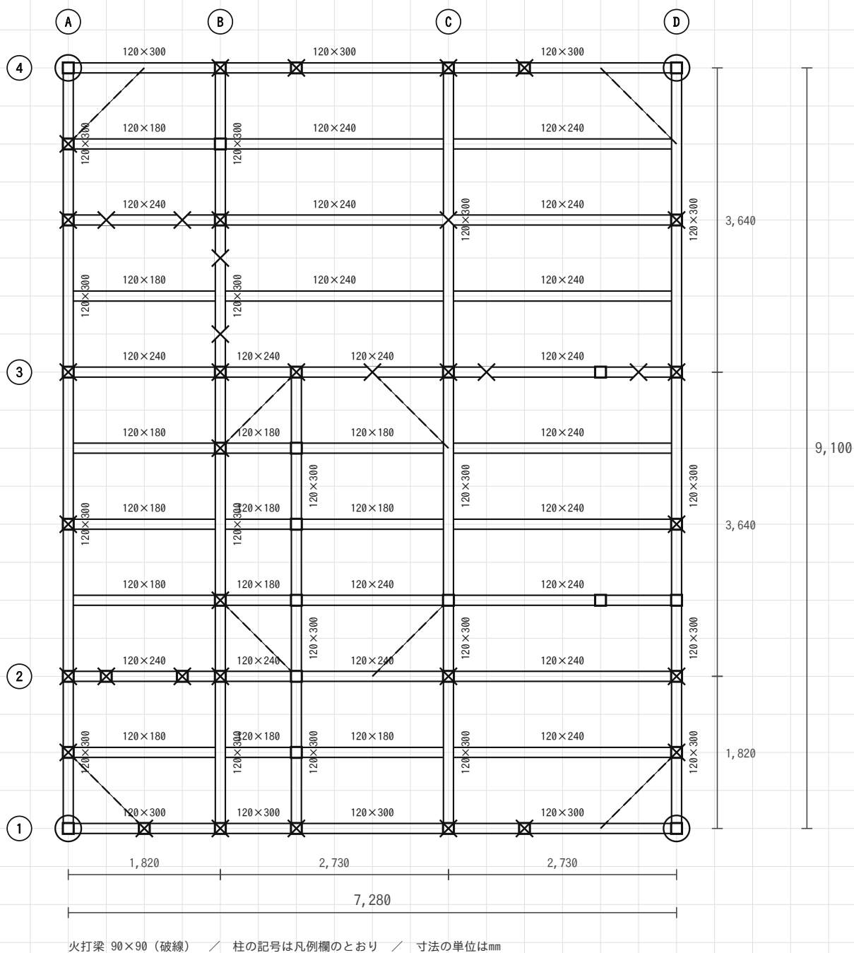
3階床伏図 縮尺1/100
