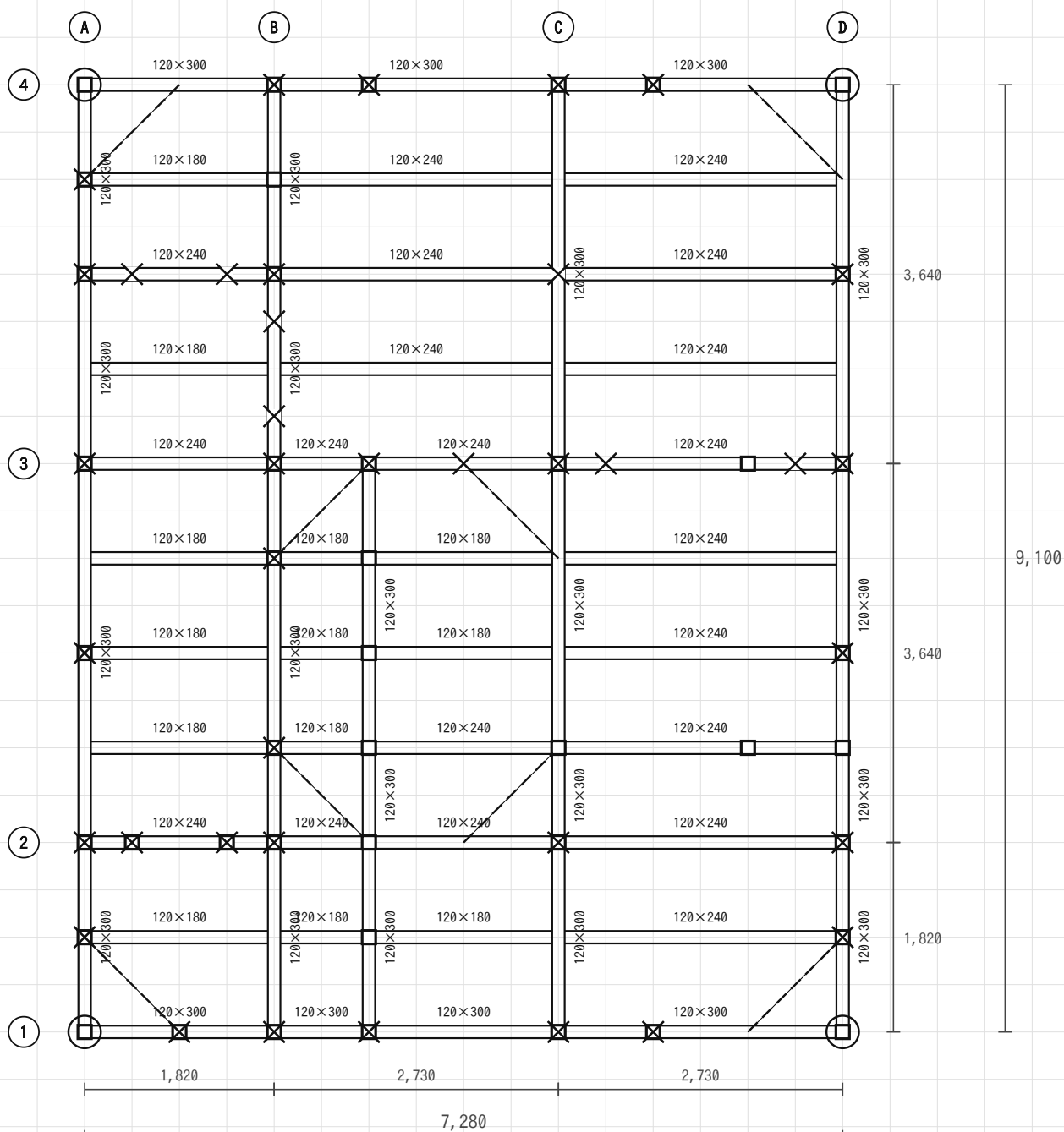
3階床伏図 縮尺1/100
