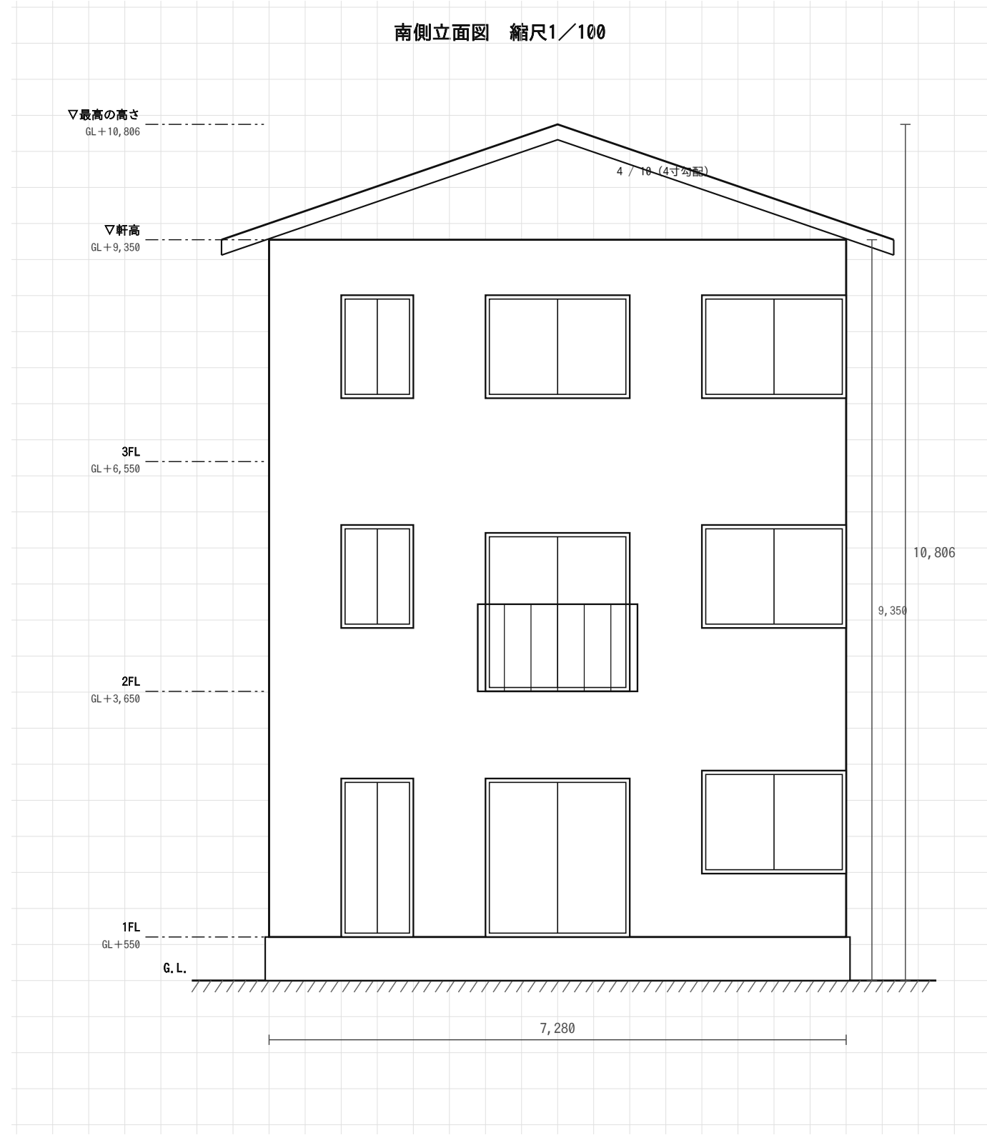
(5) 南側立面図 (1/100)
