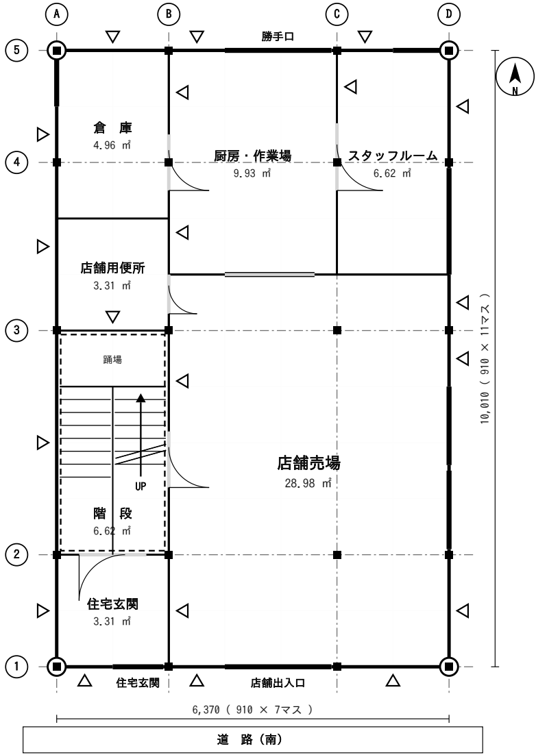
1 階平面図 兼 配置図 縮尺1／100
