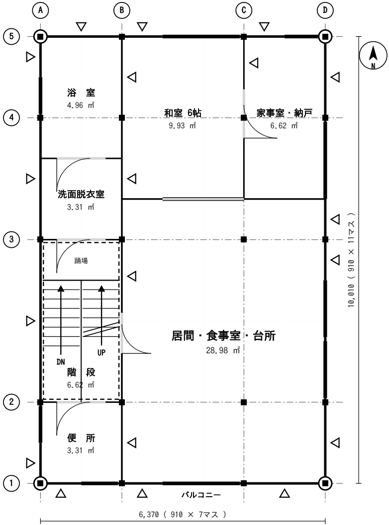
2 階平面図 縮尺1／100
