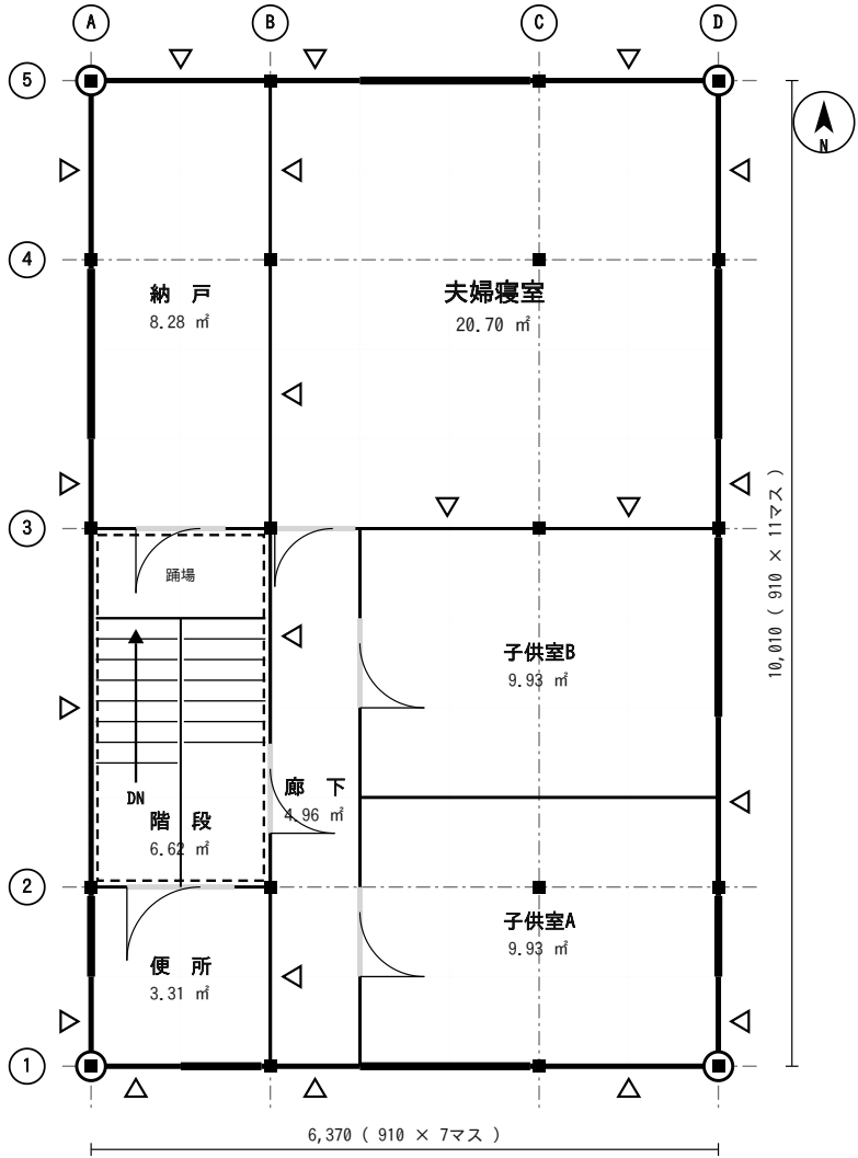
3 階平面図 縮尺1／100
