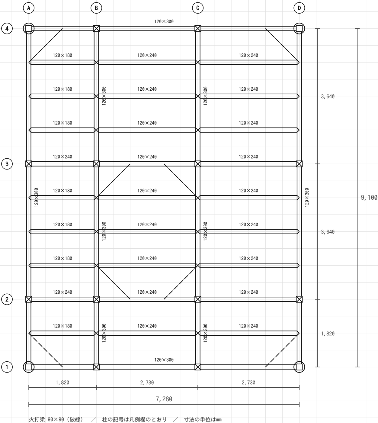
2階床伏図 兼 1階小屋伏図 縮尺1／100
