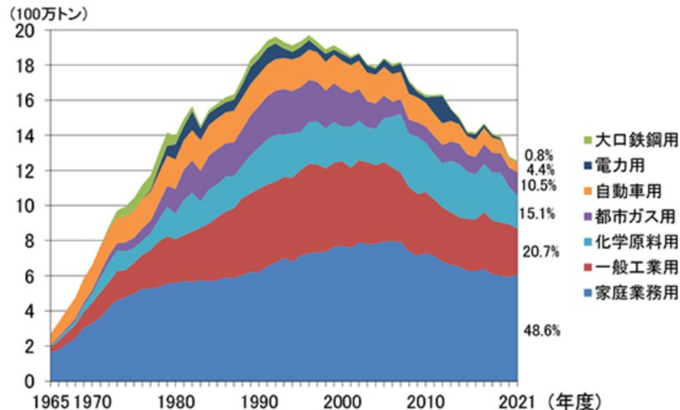
【第213-1-17】LPガスの用途別消費量の推移
