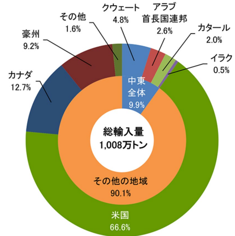
【第213-1-16】LPガスの輸入国（2021年度）
