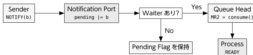
Figure 17: NOTIFY による Pending Flag の蓄積と Waiter の Wakeup
