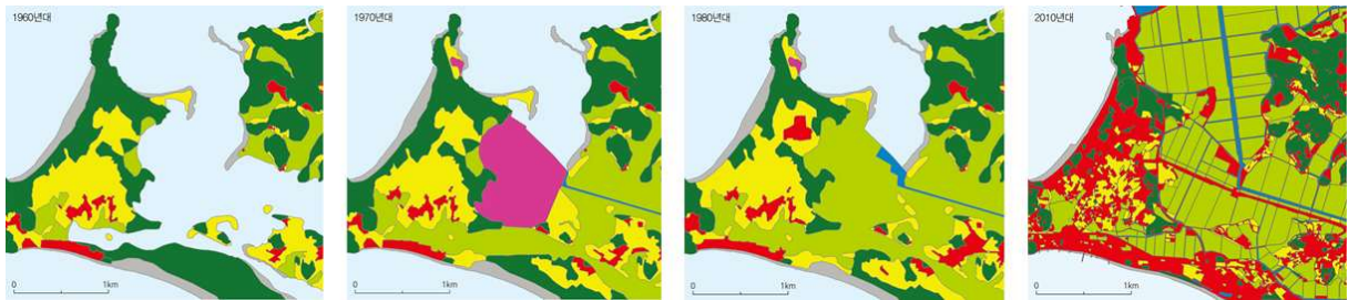
간척으로 인한 육지 면적의 변화(충남 서천군 서면)
