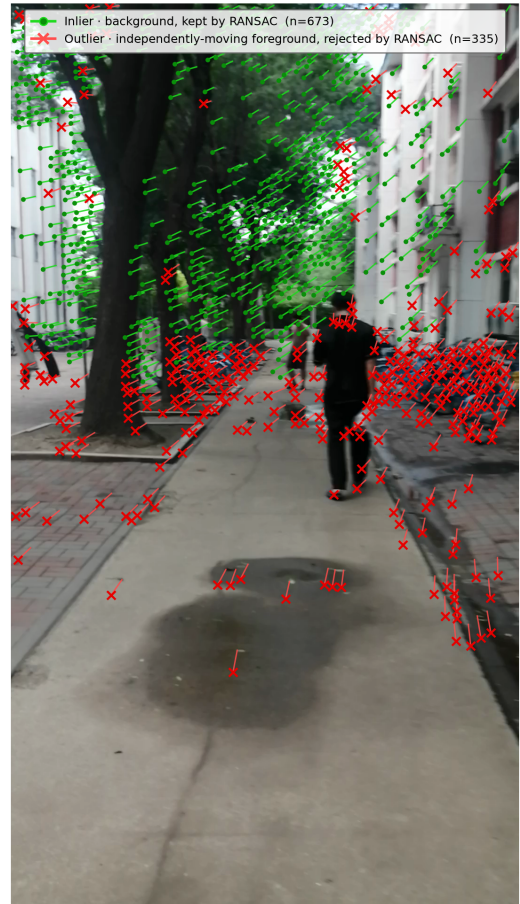
图 2 KLT 光流跟踪与外点剔除 (真实手持步行视频): 绿 = 背景内点, 红 = 被剔除的运动前景/视差点
