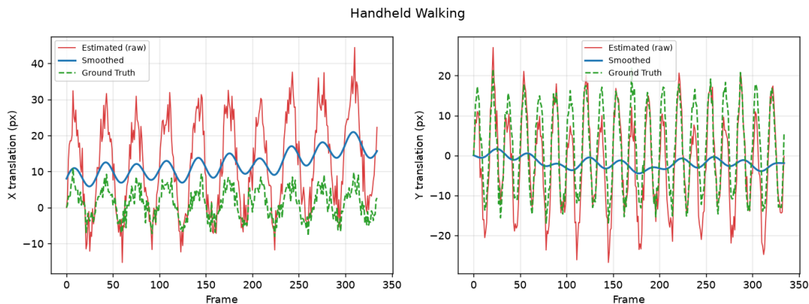
图 3 手持步行场景绝对运动轨迹对比
