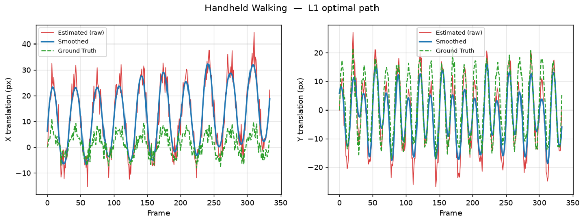
图 4 手持步行场景下 L1 最优相机路径平滑的轨迹对比
