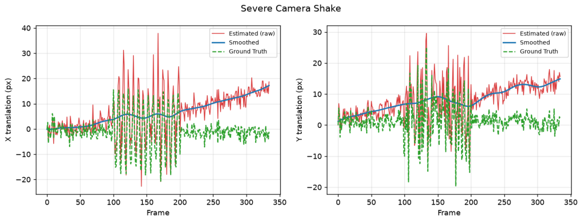
图 6 画面剧烈抖动场景绝对运动轨迹对比
