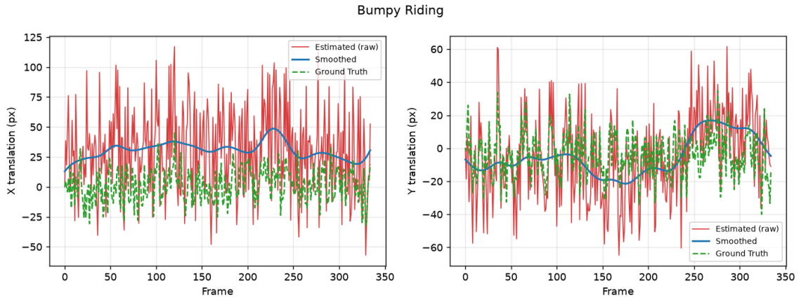
图 5 骑行颠簸场景绝对运动轨迹对比
