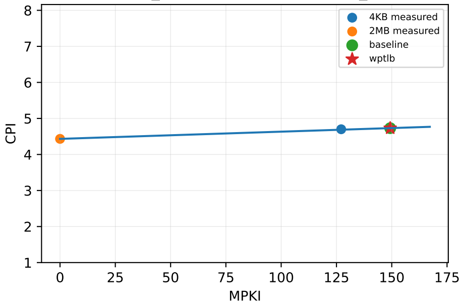
spec_cpu2017/607.cactuBSSN_s
