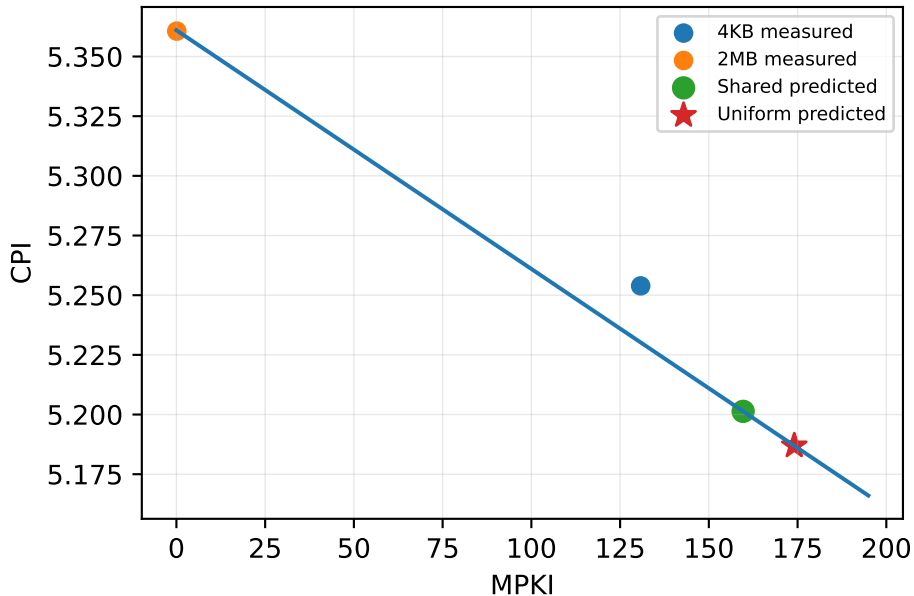
spec_cpu2017/620.omnetpp_s
