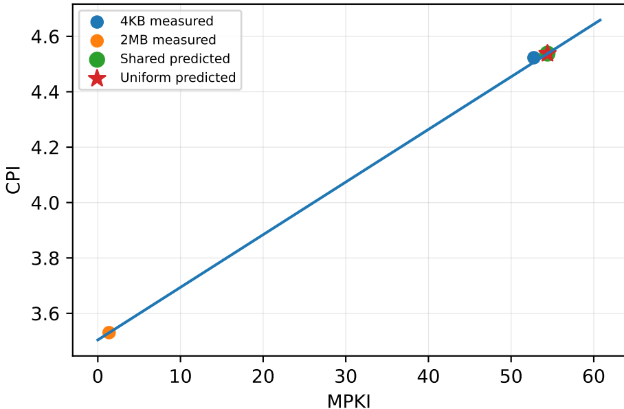
spec_cpu2017/620.omnetpp_s
