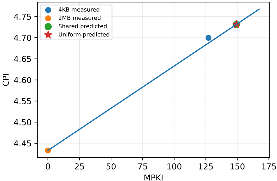
spec_cpu2017/607.cactuBSSN_s
