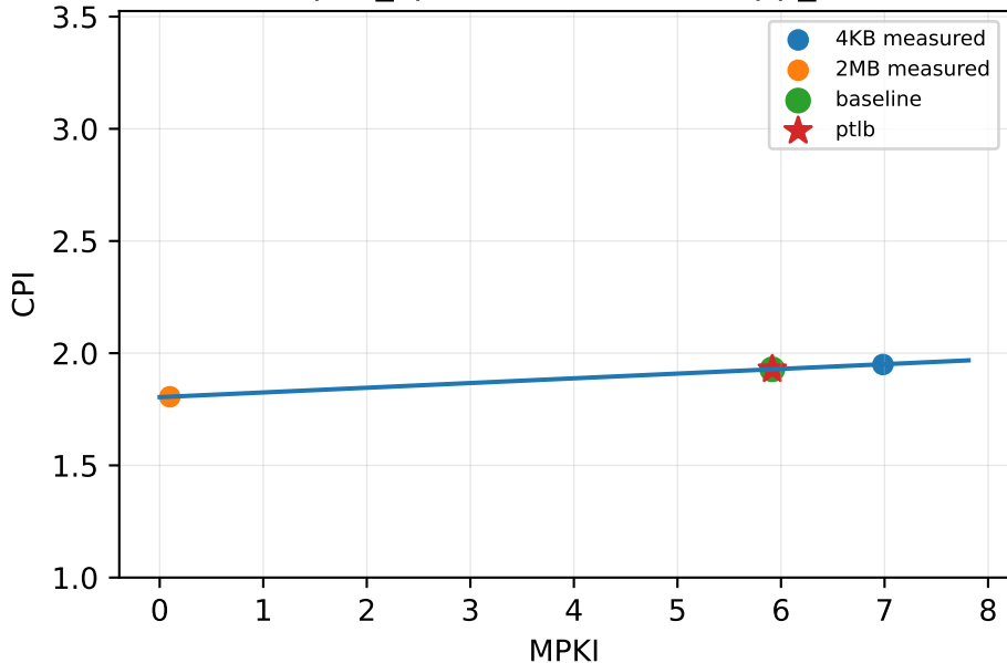
spec_cpu2017/620.omnetpp_s
