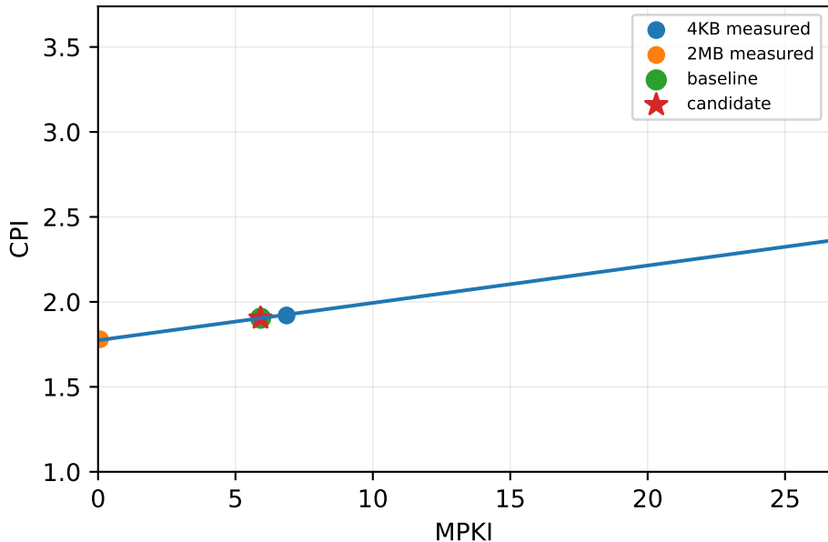
spec_cpu2017/620.omnetpp_s
