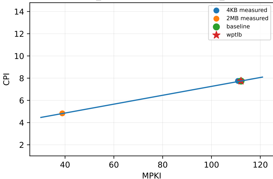
spec_cpu2017/607.cactuBSSN_s
