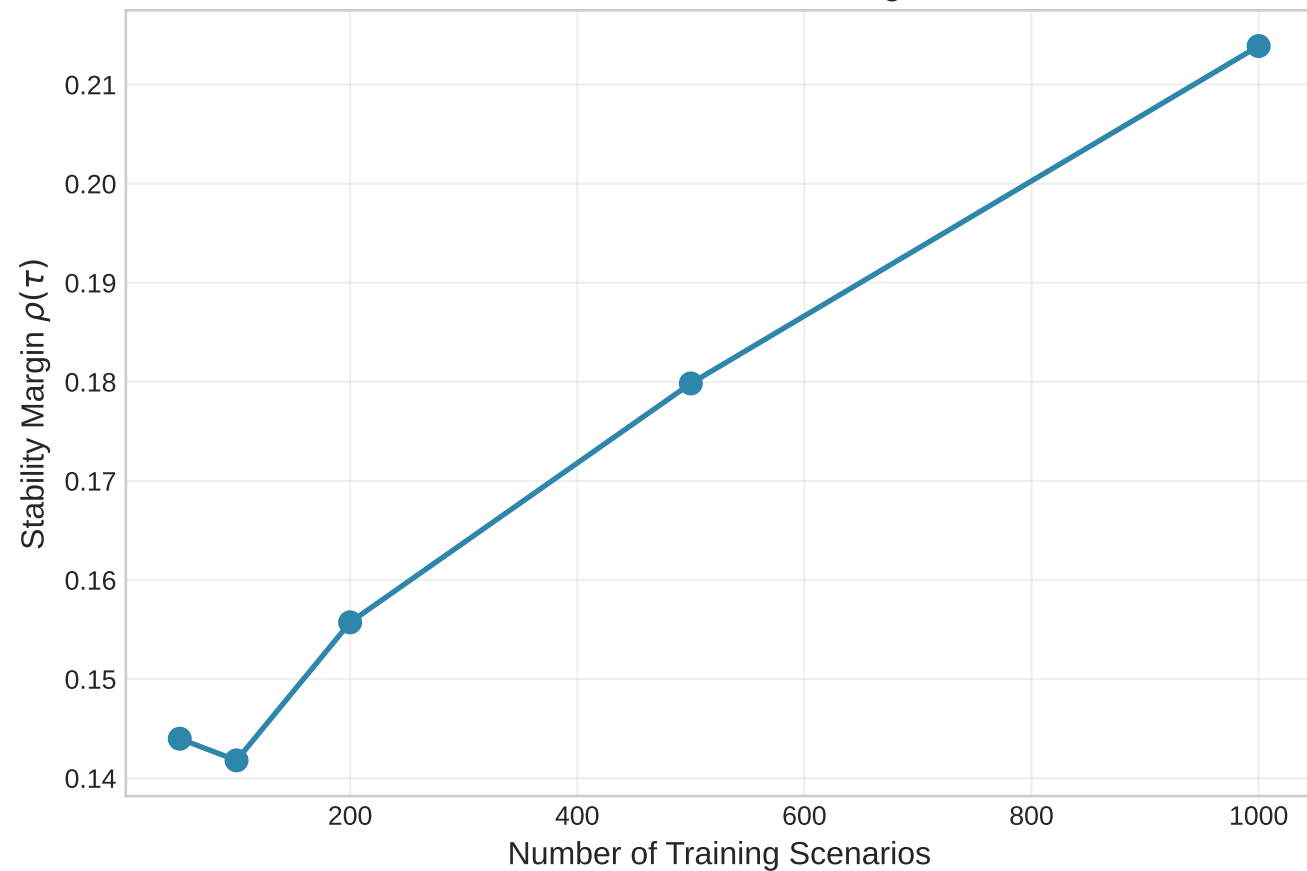
IEEE 118: Scenario Convergence
