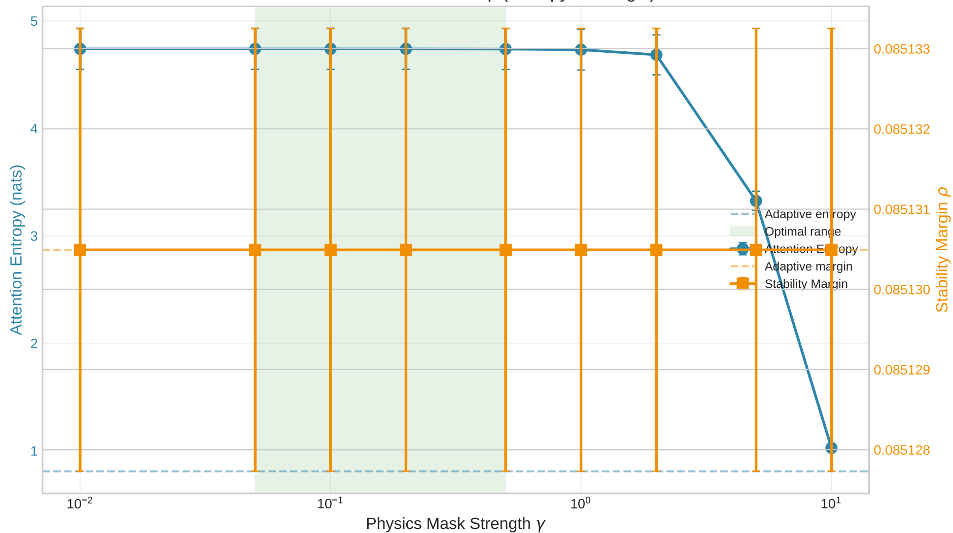
IEEE 300-Bus: Gamma Sweep (Entropy vs Margin)
