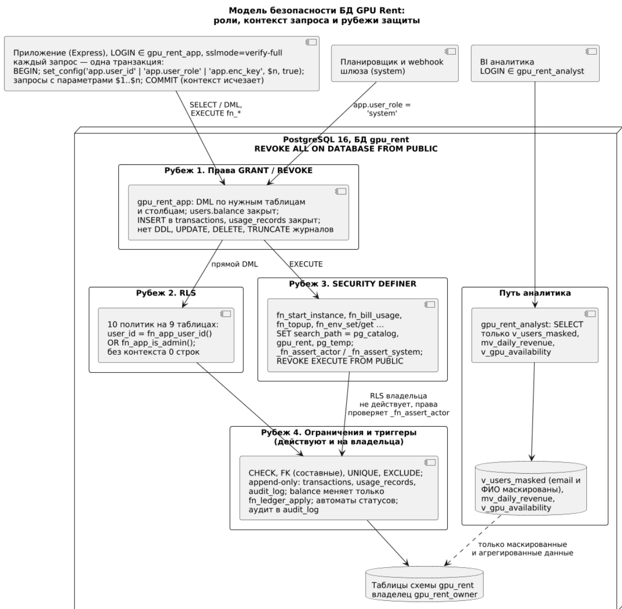
Рисунок 3 — Модель безопасности БД: роли, контекст запроса и рубежи защиты
