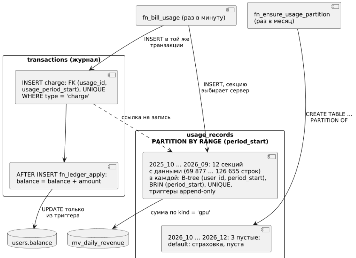
Рисунок 2 — Учёт потребления: секции usage_records и денормализованный баланс
