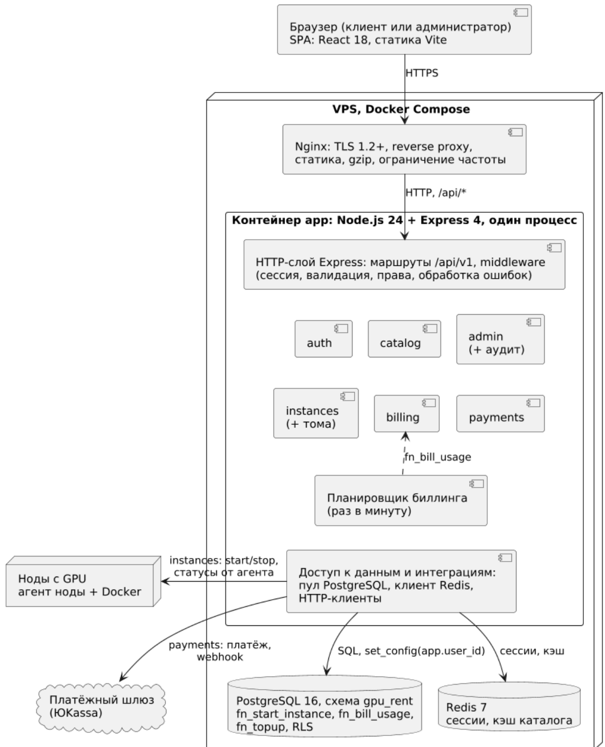
Рисунок 1 — Архитектура GPU Rent: модульный монолит
