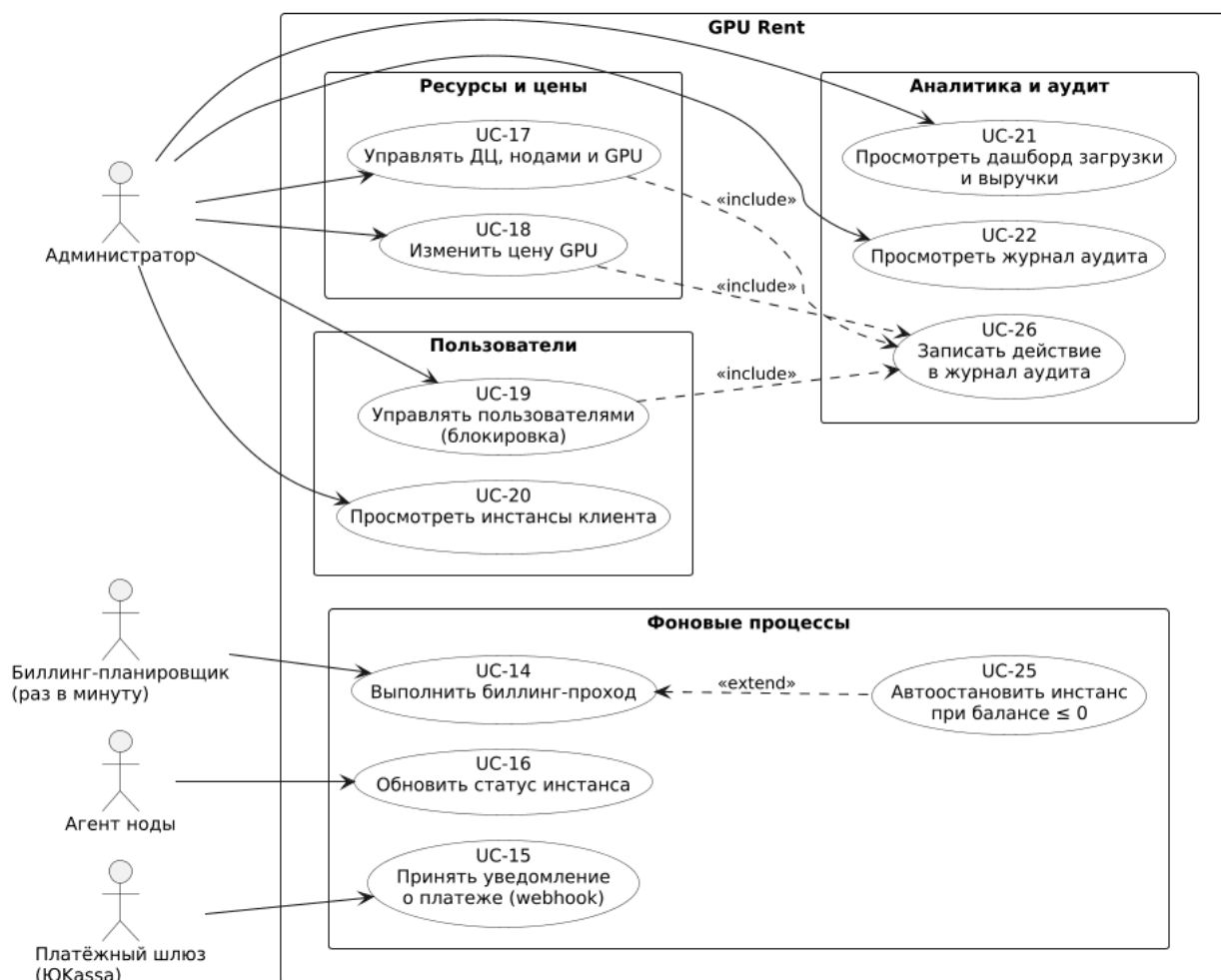
Рисунок 4 — Диаграмма вариантов использования: администратор и системные акторы
