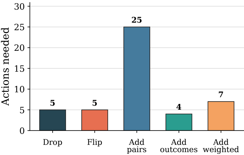
Chatbot Arena 55k (k=5)
