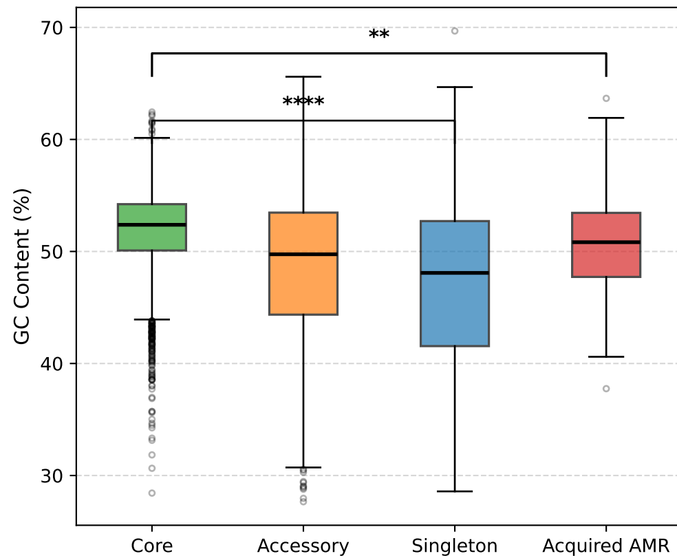
A) Gene GC Content
