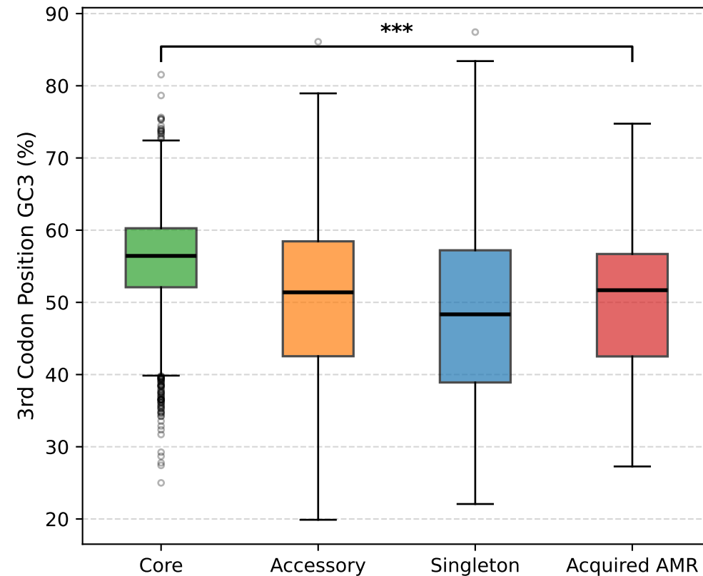
B) Codon Bias (GC3)
