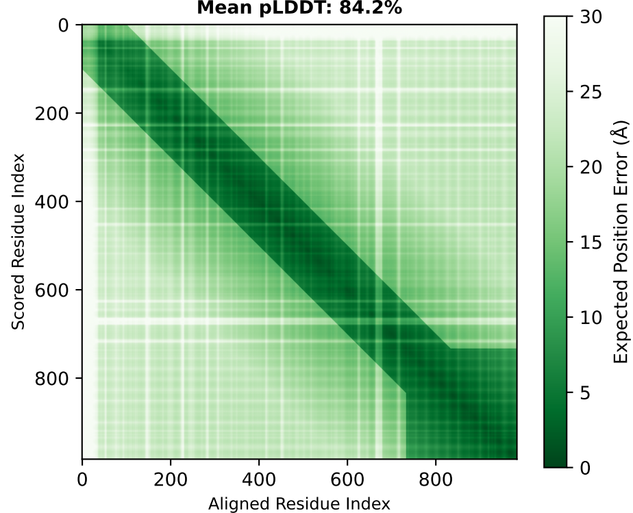
(d) OAT_371 (KNGPFPPJ_04371) Mean pLDDT: 84.2%
