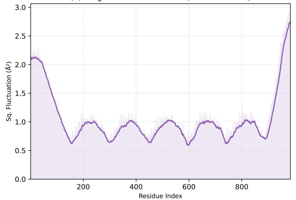
(d) OAT_371 — ANM Modes 7-9 (n=984 residues)
