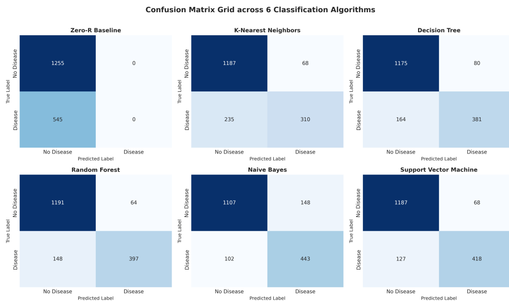
Figure 2: Grille des Matrices de Confusion des 6 Algorithmes Benchmarkés.
