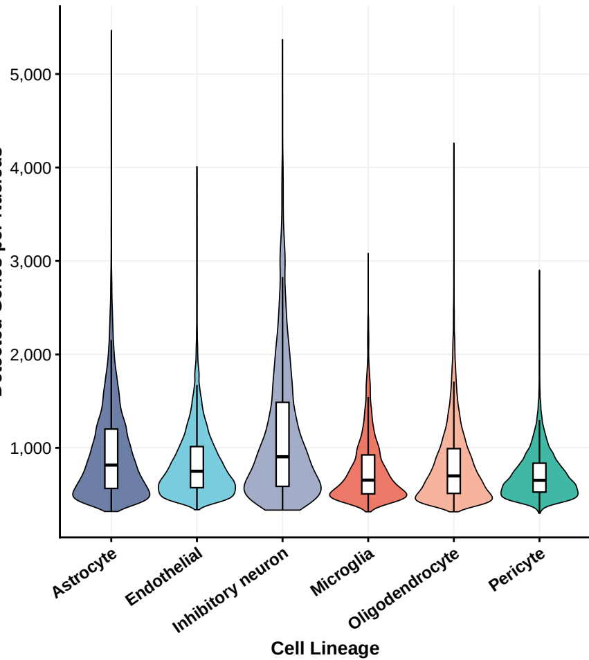
Detected Genes per Nucleus
