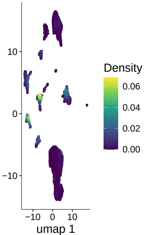
Ppargc1a
