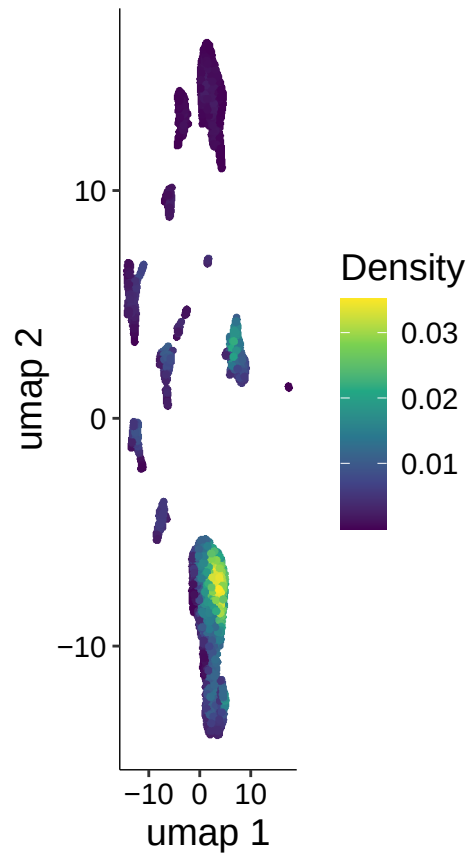
Phlda3
