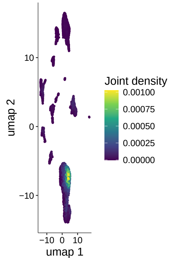
Ccnd1+ Phlda3+
