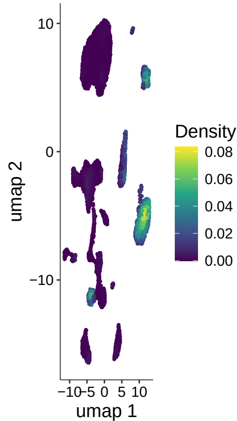
Phlda3
